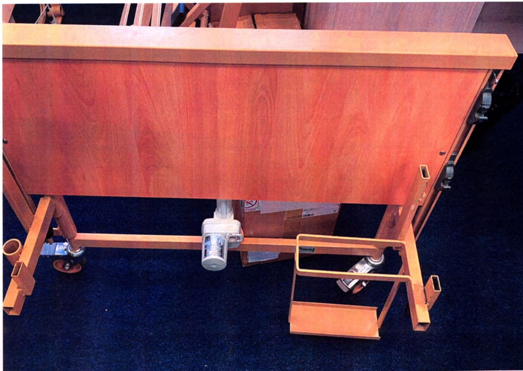
Изножье деревянное в сборе «Кровать медицинская функциональная электрическая Burmeister с принадлежностями, в вариантах исполнения: Dali Standard, Dali Standard Econ, Dali Low Entry, Dali Low Entry Econ»
