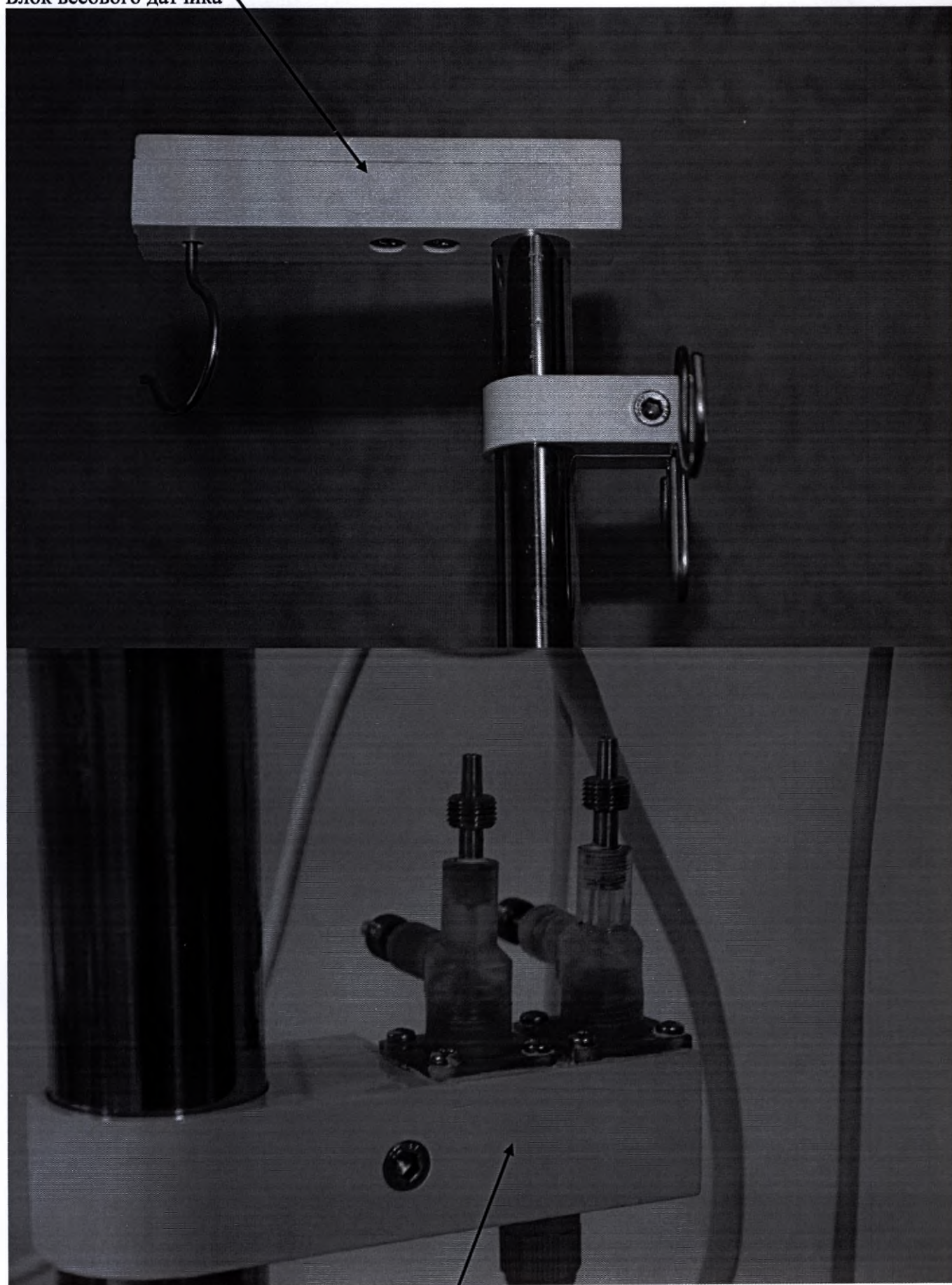
Блок весового датчика
