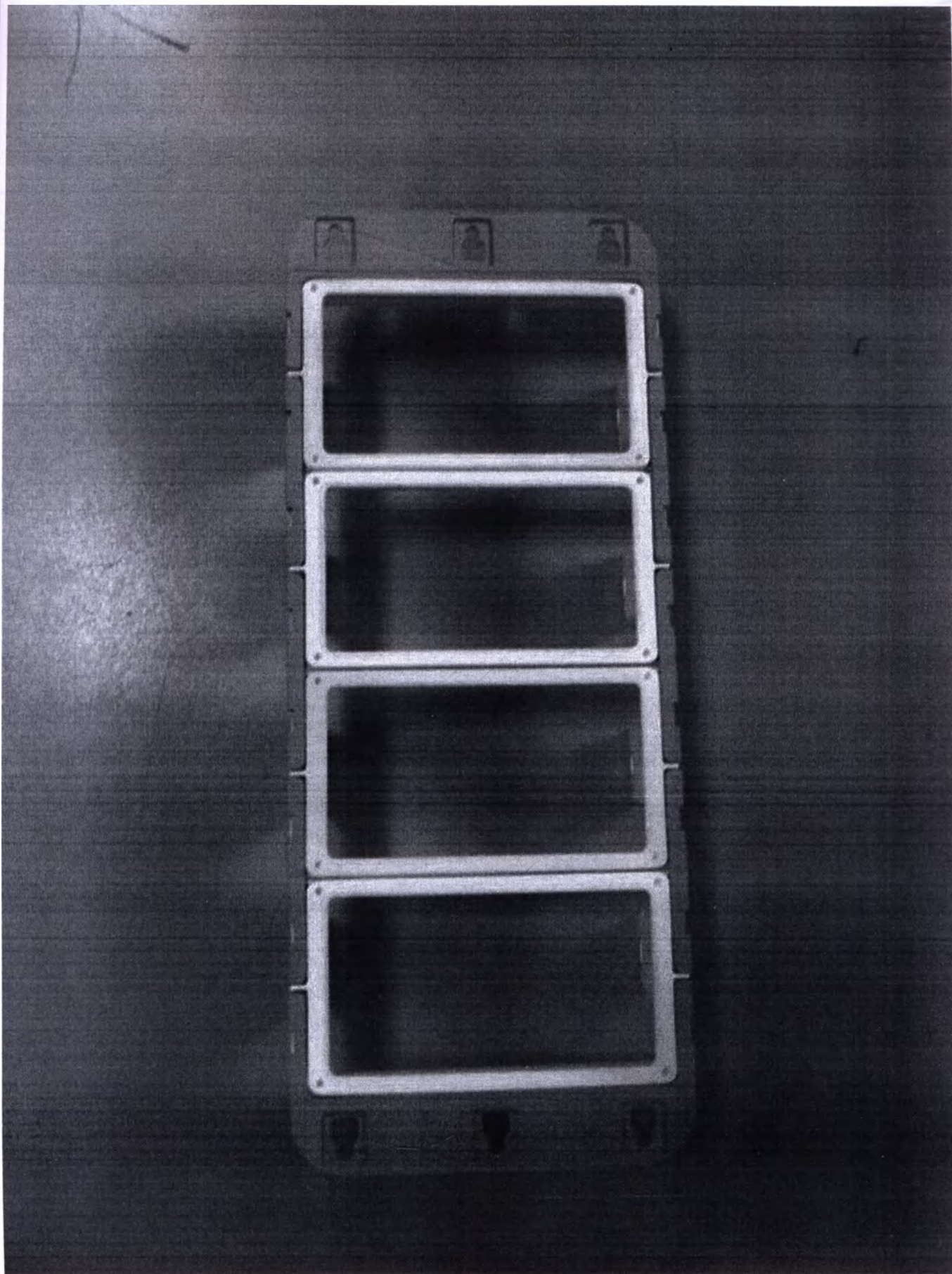
Рамка для крепления манипулы 40х60 на 4 ячейки
