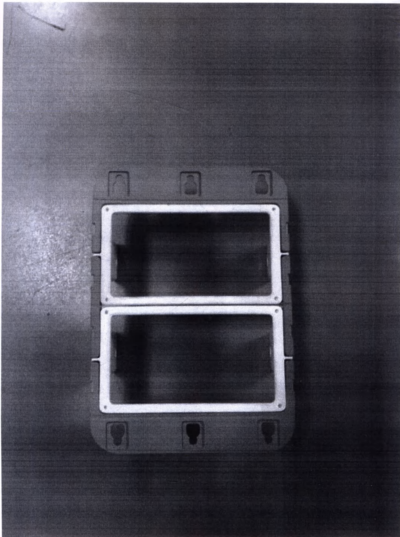
Рамка для крепления манипулы 40x80 на 2 ячейки по широкой части
