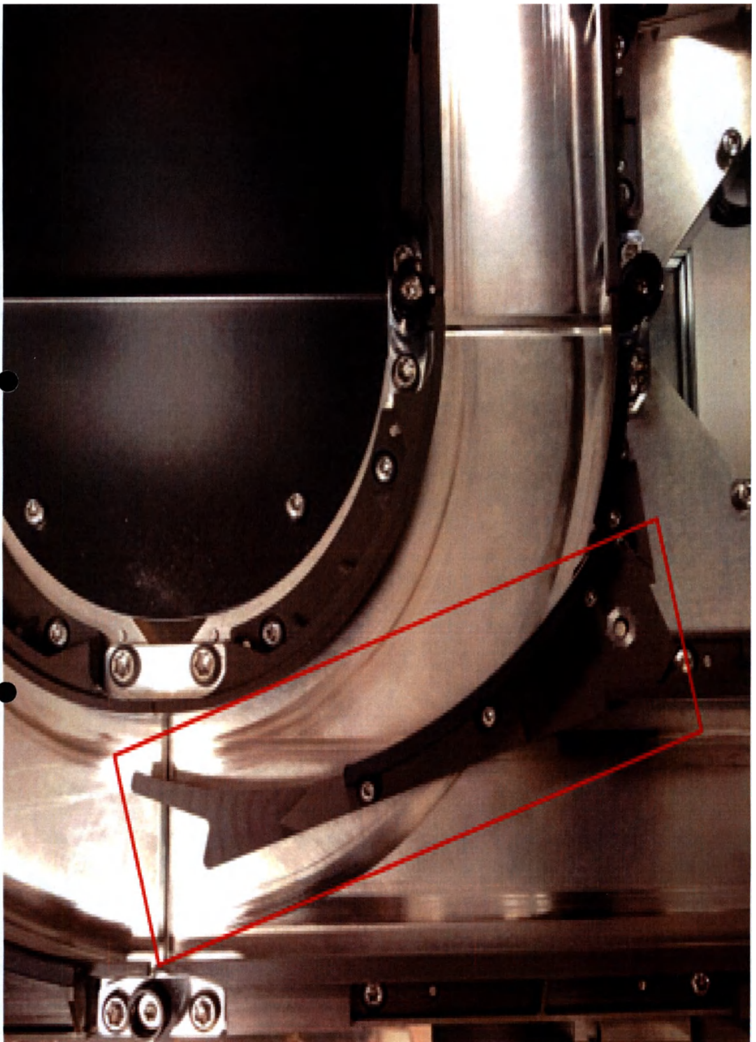
3.5. Переключатели линии транспортировочной левые
