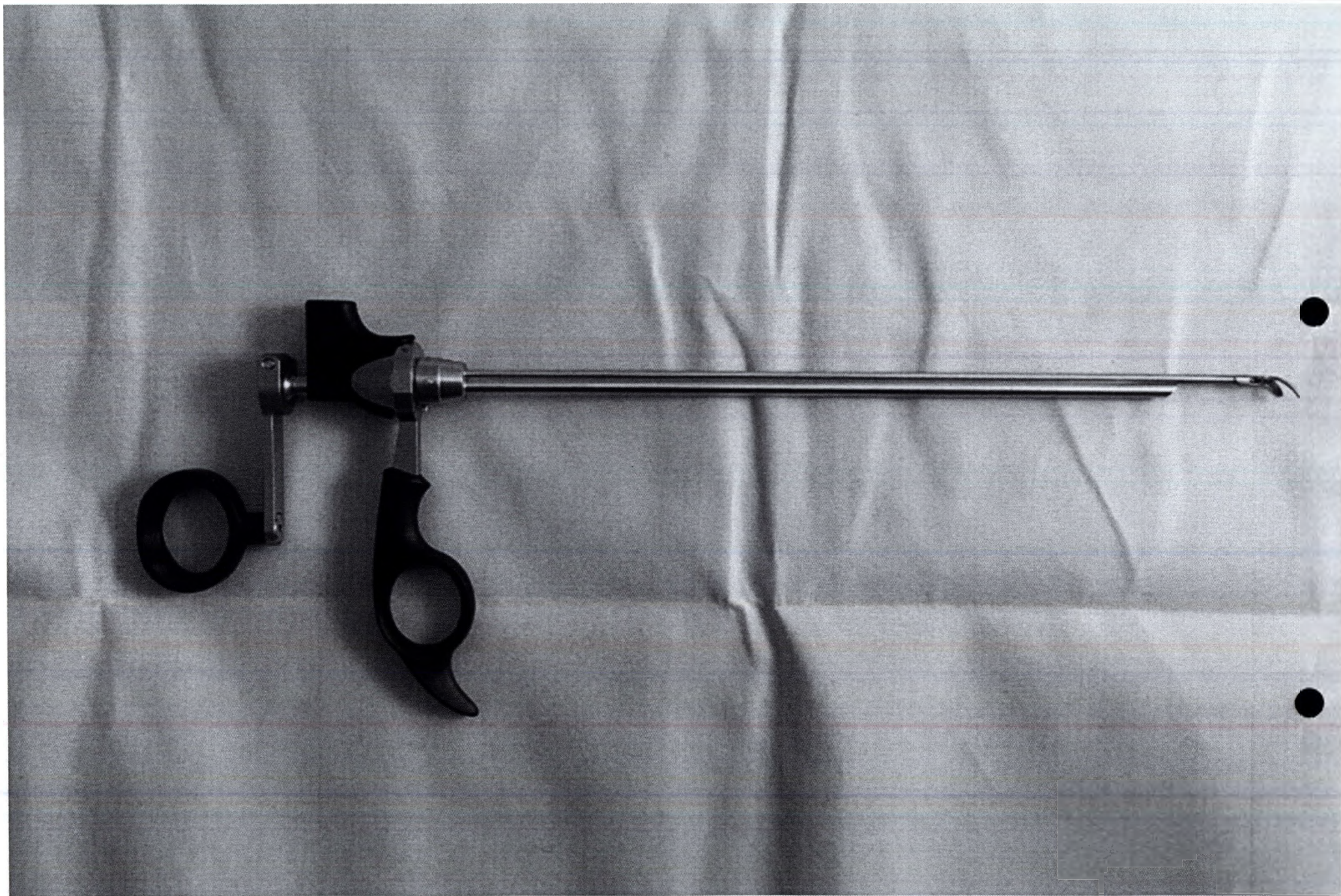
Ножницы, оптические: A4678, A20717A.
