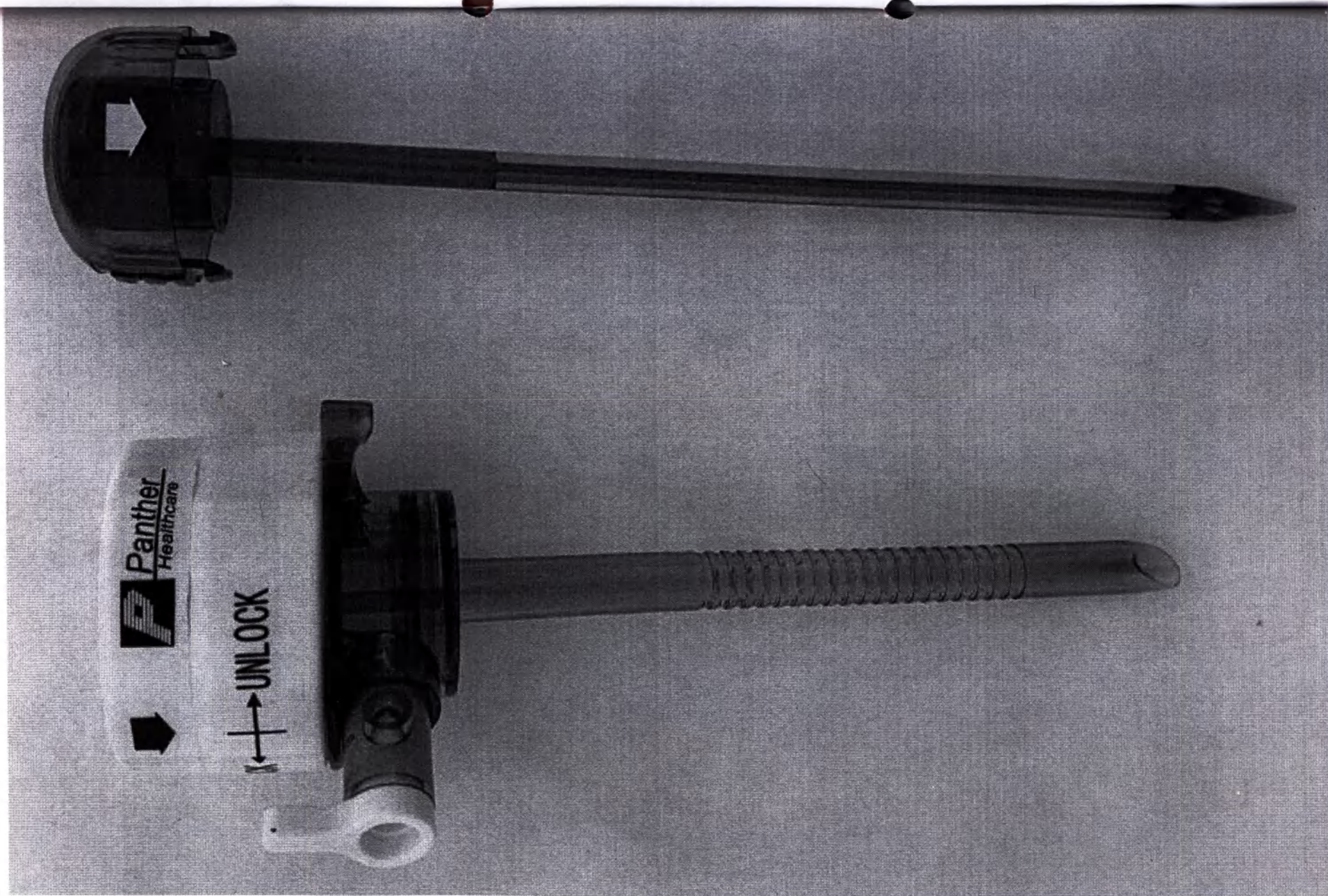
Рис. 1 Троакар хирургический одноразовый, безлезвийный с канюлей, PBS051R1, диаметр 5 мм, длина 110 мм – общий вид изделия
