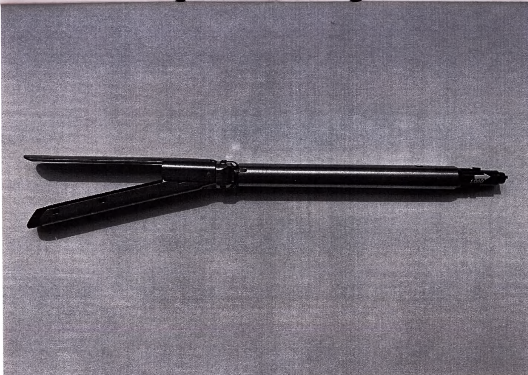
Рис. 12 Кассеты сменные, артикуляционные со скобами и ножом для степлера сшивающего хирургического, эндоскопического, CADF-60R, длина 60 мм, высота скоб 5,0 мм – общий вид
