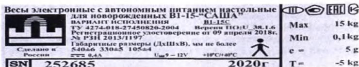
Рисунок 5.1 – Планка фирменная (образец)
