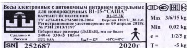
Рисунок 5.1 – Планка фирменная (образец)
