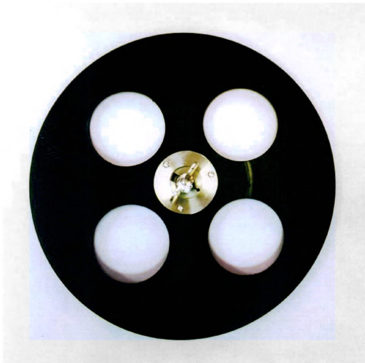
Верхний диск револьверного держателя кювет
