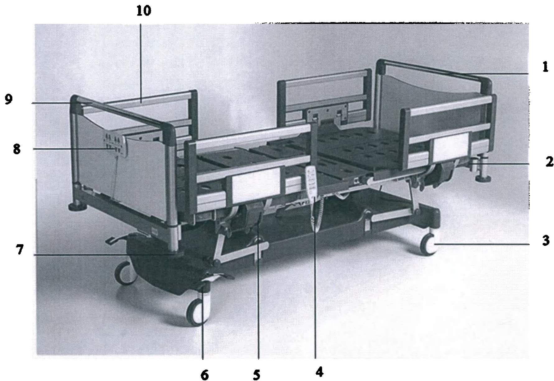
1. Панель изголовья. 2. Рычаг CPR. 3. Колеса Ø 125 мм. 4. Пульт управления ручной. 5. Механизм открытия/закрытия бокового ограждения. 6. Система центральной блокировки колес. 7. Бампер защитный. 8. Панель управления для медицинского персонала. 9. Панель изножья. 10. Ограждение боковое
