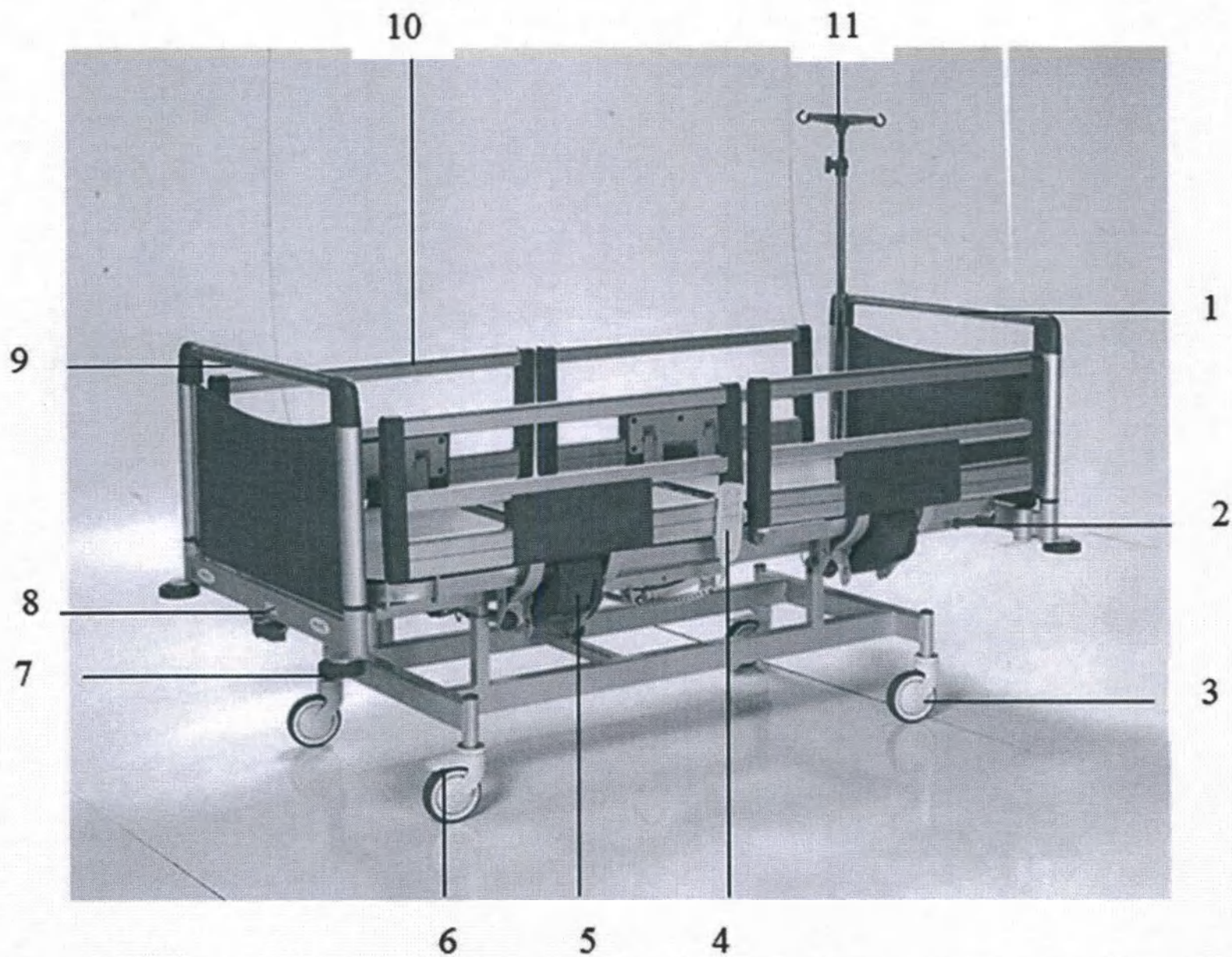
1. Панель изголовья. 2. Рычаг CPR. 3. Колеса Ø 125 мм. 4. Пульт управления ручной. 5. Механизм открытия/закрытия бокового ограждения. 6. Система блокировки колес. 7. Бампер защитный. 8. Рычаг положения Тренделенбурга. 9. Панель изножья. 10. Ограждения боковые. 11. Инфузионная стойка
