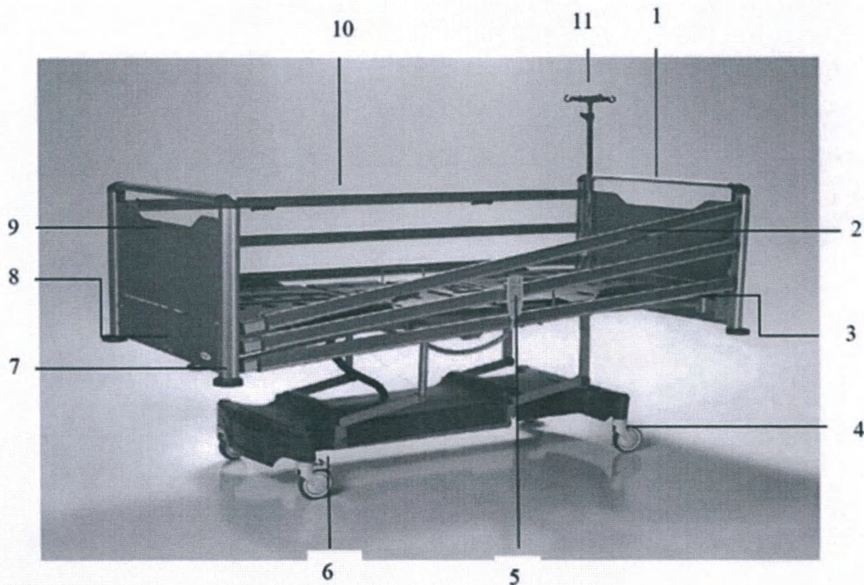
1. Панель изголовья. 2. Механизм открытия/закрытия бокового ограждения. 3. Рычаг CPR. 4. Колесо Ø125 мм. 5. Пульт управления ручной. 6. Система блокировки колес. 7. Бампер защитный. 8. Регулировка положения Тренделенбурга. 9. Панель изножья. 10. Ограждение боковое. 11. Инфузионная стойка
