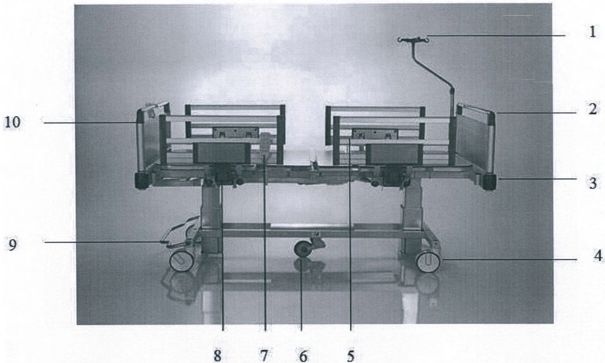
1. Инфузионная стойка. 2. Панель изголовья. 3. Бампер защитный. 4. Колеса Ø 150 мм . 5. Ограждение боковое 6. 5-е колесо. 7. Пульт управления ручной. 8. Блокировка открытия/закрытия бокового ограждения. 9. Система центральной блокировки колёс. 10. Панель изножья
