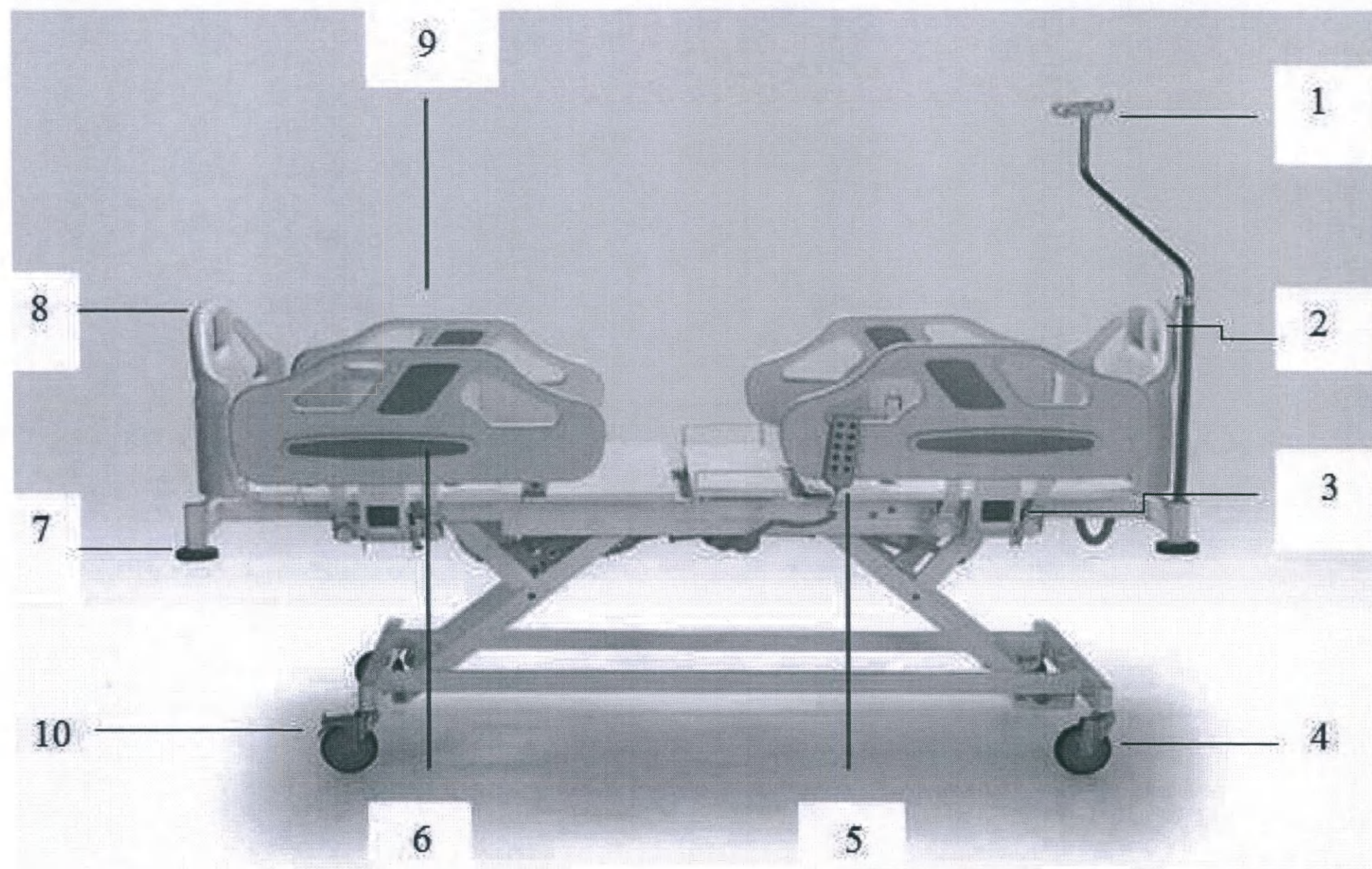
1. Стойка инфузионная. 2. Панель изголовья. 3. Блокировка открытия/закрытия бокового ограждения. 4. Колеса Ø125 мм. 5. Пульт управления ручной. 6,9. Ограждения боковые. 7. Бампера защитные. 8. Панель изножья. 10. Педаль перекрестной блокировки колес
