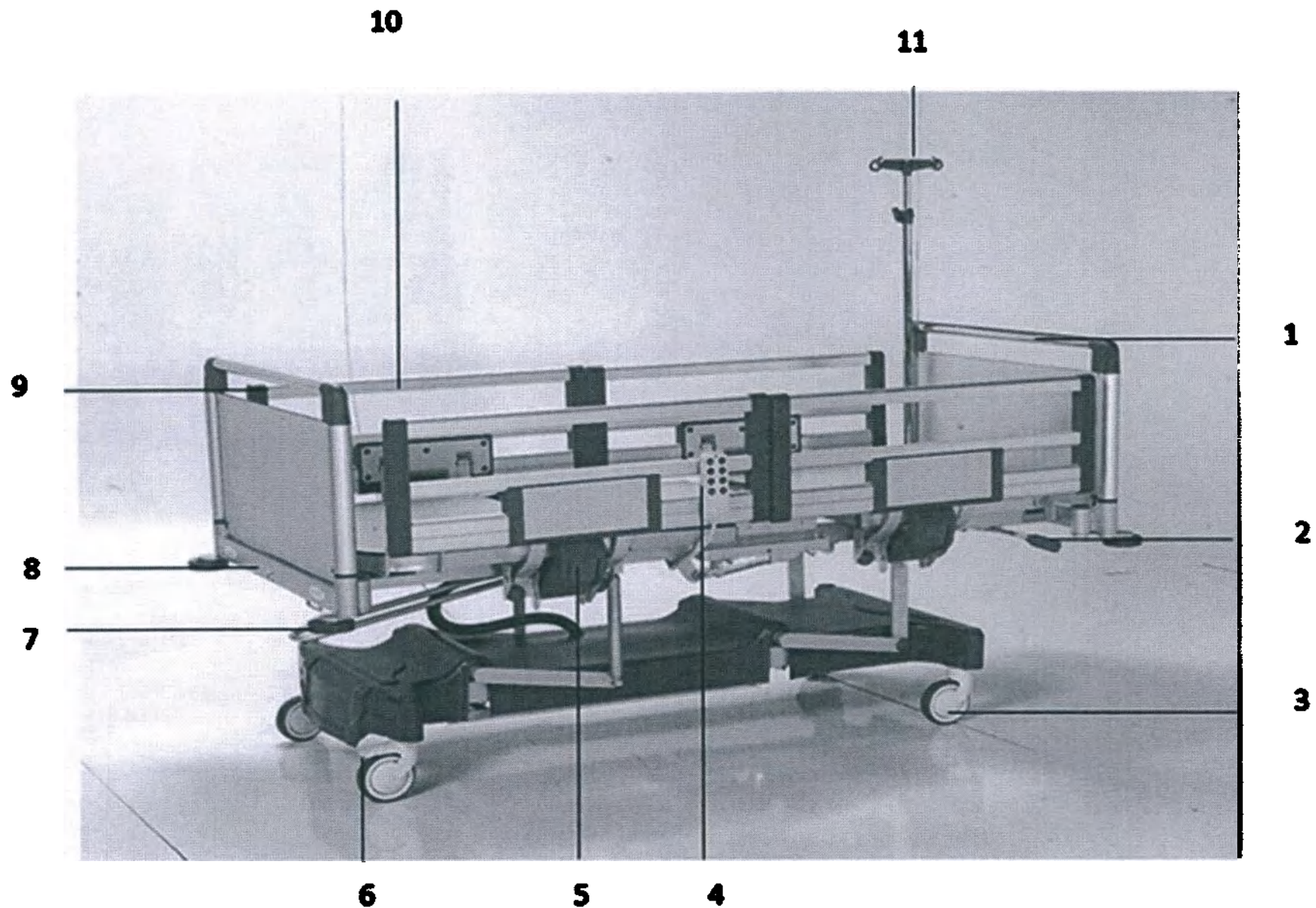
1. Панель изголовья. 2. Рычаг CPR. 3. Колеса Ø 125 мм. 4. Пульт управления ручной. 5. Механизм открытия/закрытия бокового ограждения. 6. Система блокировки колес. 7. Бампер защитный. 8. Рычаг положения Тренделенбурга. 9. Панель изножья. 10. Ограждение боковое. 11. Инфузионная стойка
