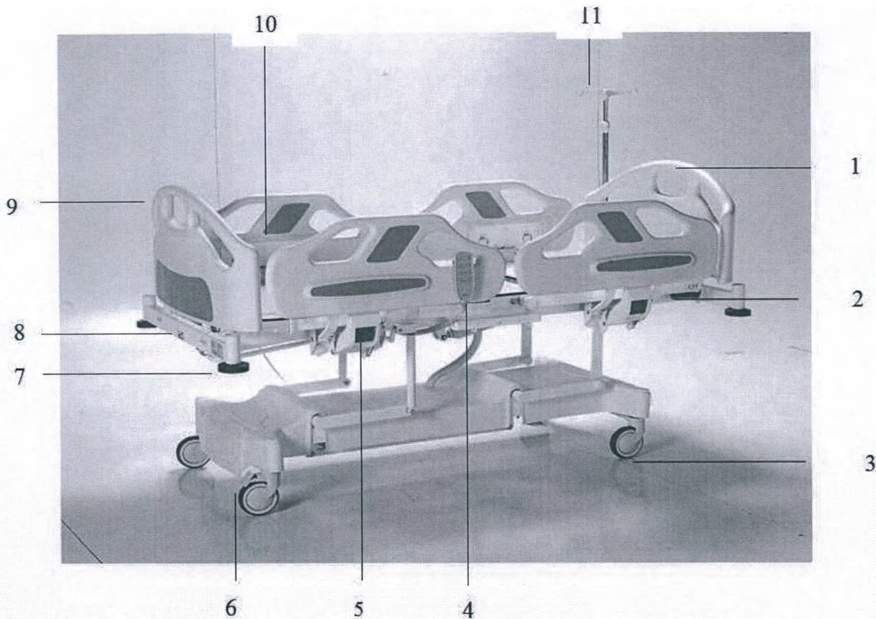
1. Панель изголовья. 2. Рычаг CPR. 3. Колеса Ø125 мм. 4. Пульт управления ручной. 5. Блокировка бокового ограждения. 6. Система блокировки колес. 7. Бампер защитный. 8. Регулировка положения Тренделенбурга. 9. Панель изножья. 10. Ограждения боковые. 11. Инфузионная стойка
