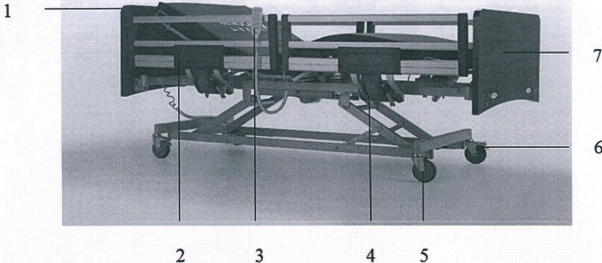
1. Панель изголовья. 2. Ограждение боковое. 3. Пульт управления ручной. 4. Рычаг открытия/закрытия бокового ограждения. 5. Колесо Ø125 мм. 6. Система перекрестной блокировки колес. 7. Панель изножья
