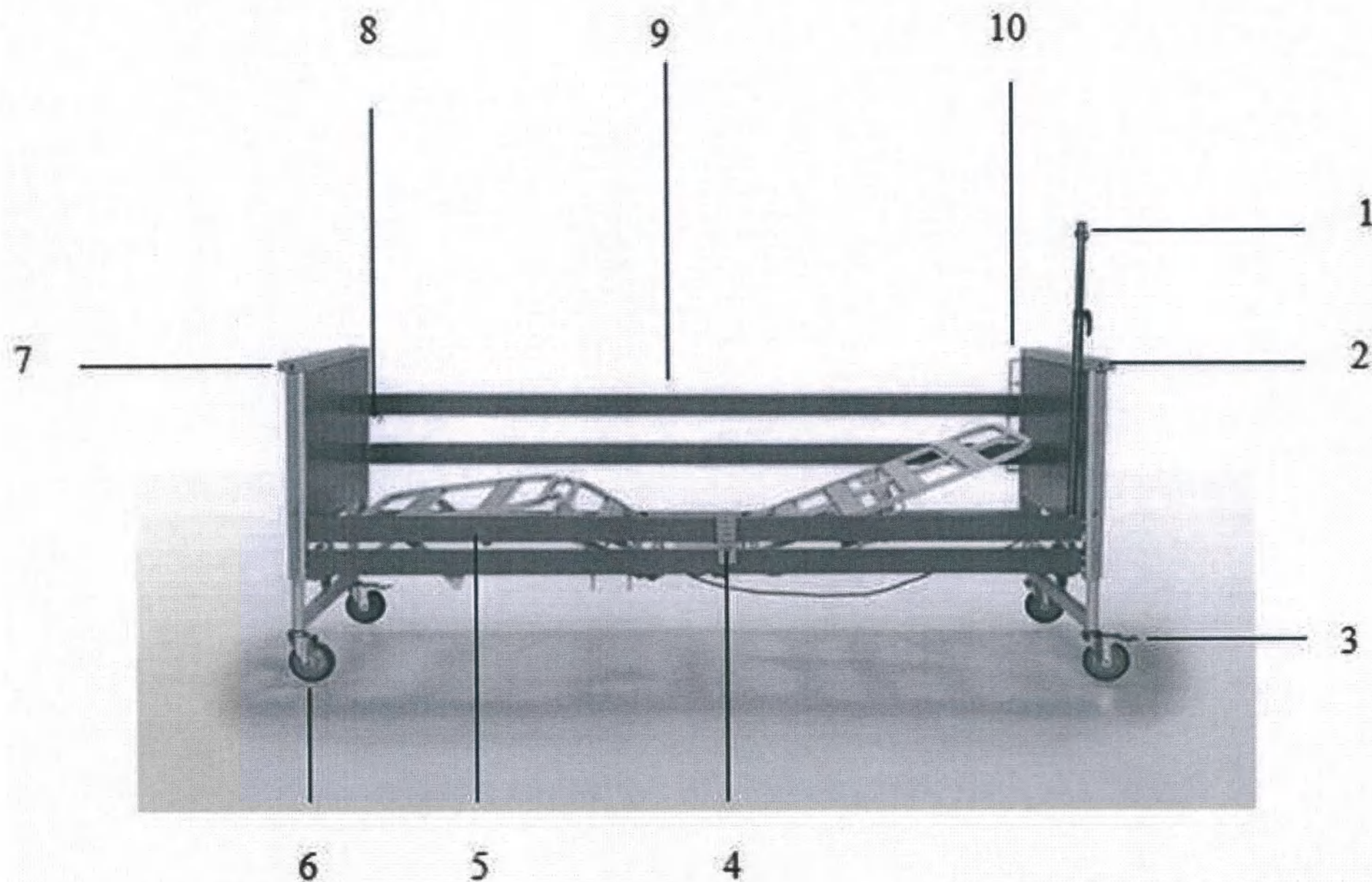
1. Инфузионная стойка. 2. Панель изголовья. 3. Система блокировки колес. 4. Пульт управления ручной. 5. Боковое ограждение. 6. Колесо Ø125 мм. 7. Панель изножья. 8. Механизм открытия/закрытия бокового ограждения. 9. Боковое ограждение. 10. Держатель для кислородной трубки
