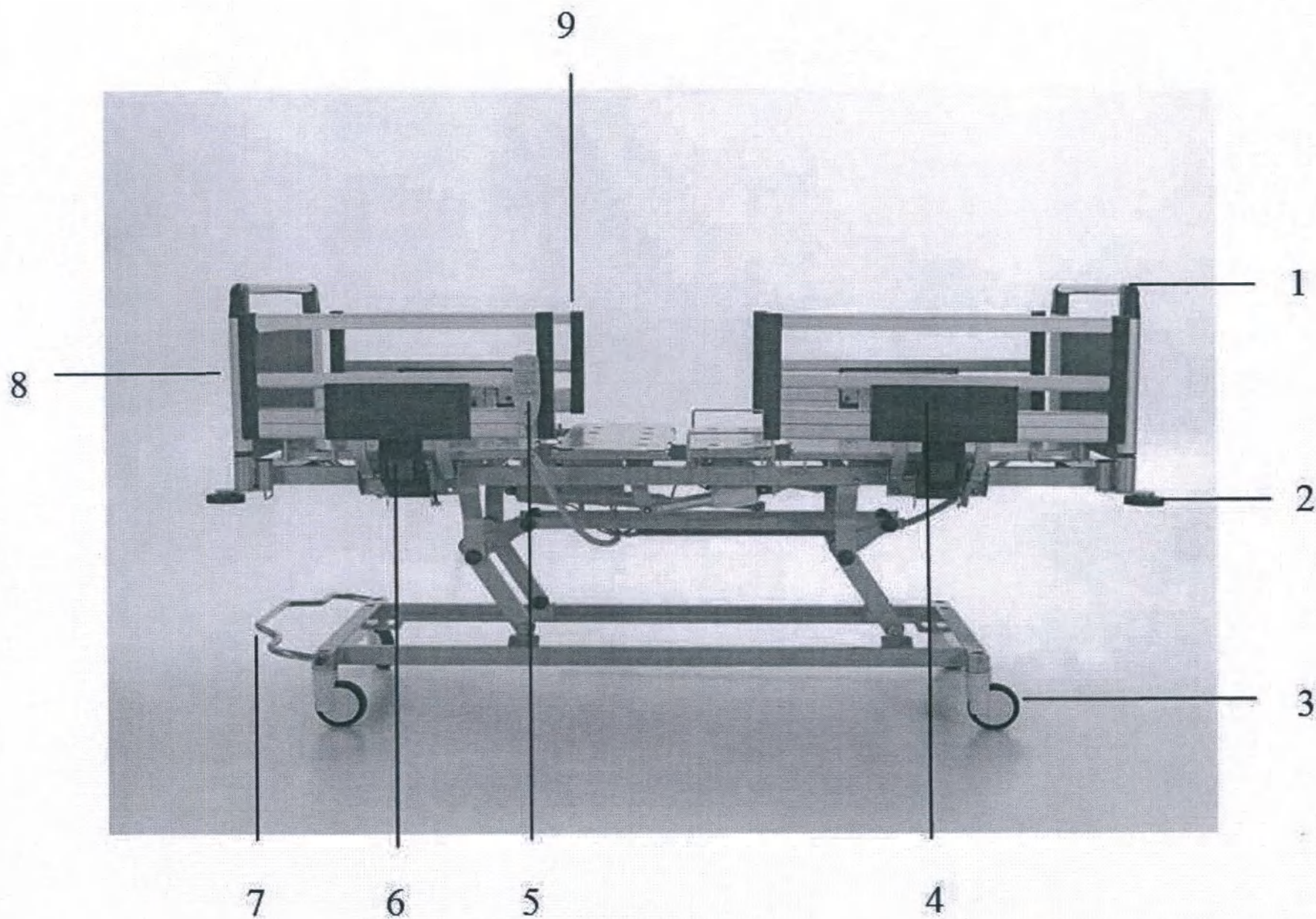
1. Панель изголовья. 2. Бампер защитный. 3. Колесо Ø125 мм. 4,9. Ограждение боковое. 5. Пульт управления ручной. 6. Механизм открытия/закрытия бокового ограждения. 7. Система центральной блокировки колес. 8. Панель изножья
