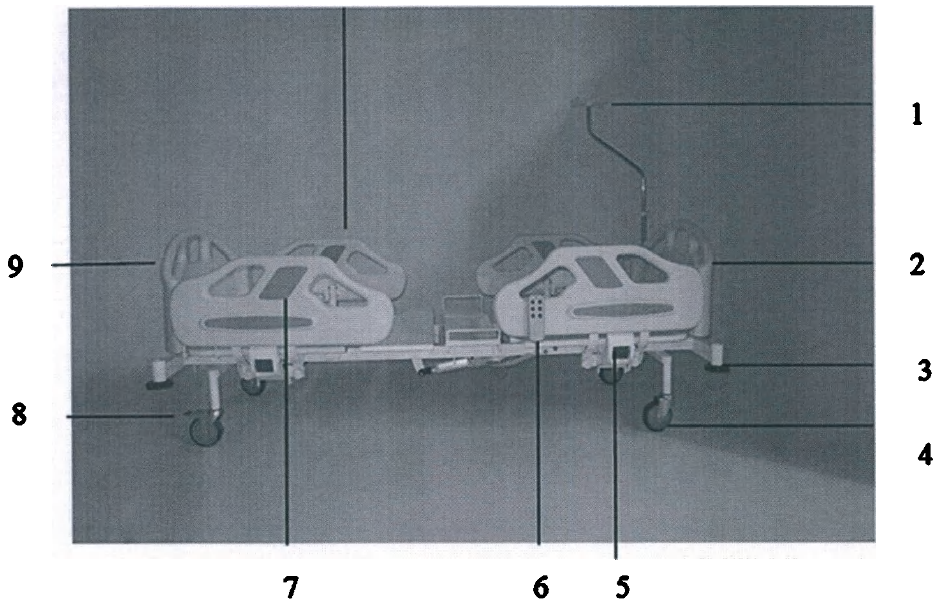
1. Инфузионная стойка. 2. Панель изголовья. 3. Бампер защитный. 4. Колеса Ø125 мм. 5. Механизм открытия/закрытия бокового ограждения. 6. Пульт управления. 7. Ограждение боковое. 8. Система перекрестной блокировки колес. 9. Панель изножья. 10. Ограждение боковое
