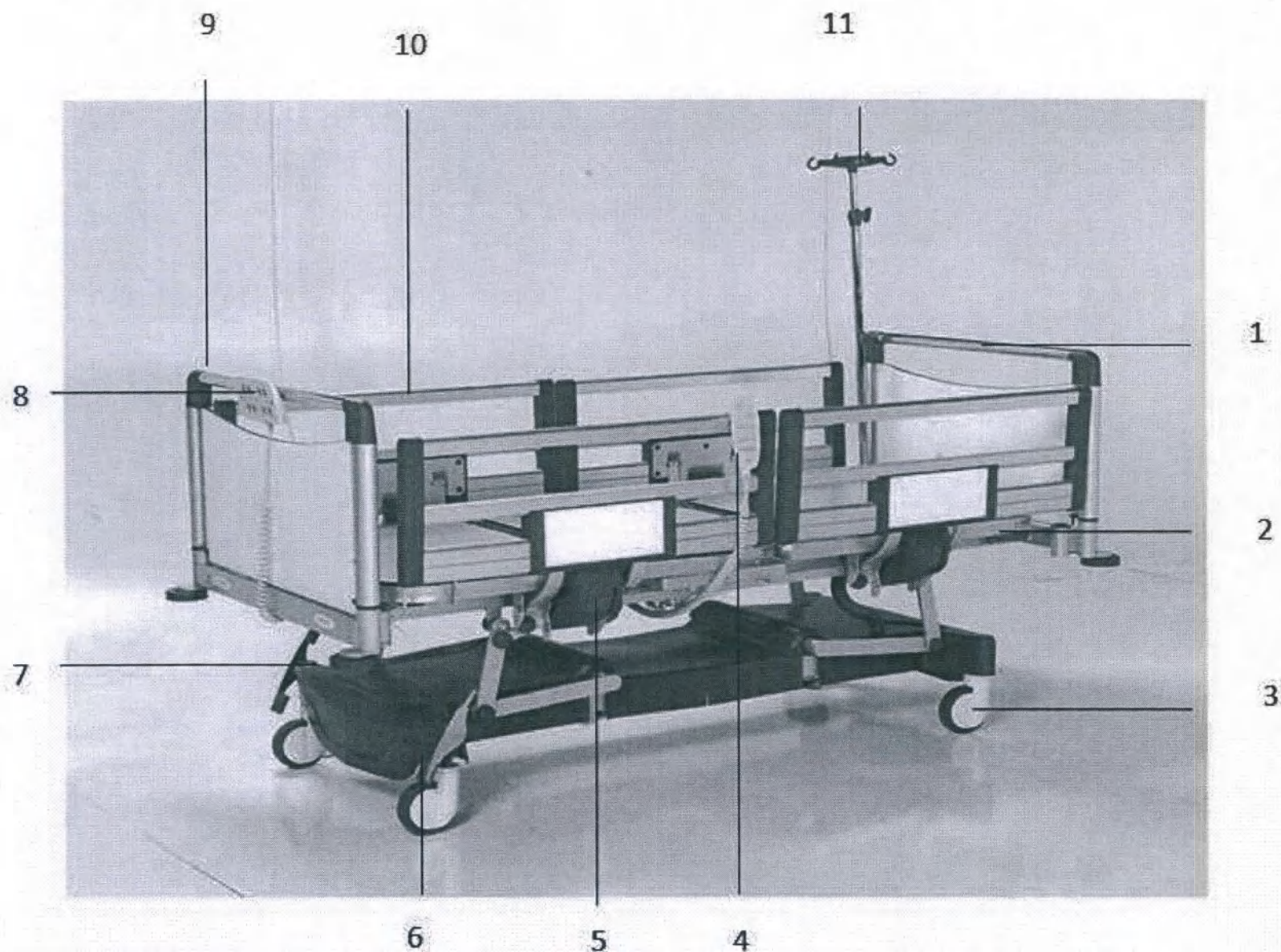
1. Панель изголовья. 2. Рычаг CPR. 3. Колеса Ø 125 мм. 4. Пульт управления ручной. 5. Механизм открытия/закрытия бокового ограждения. 6. Система блокировки колес центральная. 7. Бампер защитный. 8. Панель управления для медицинского персонала. 9. Панель изножья. 10. Ограждение боковое. 11. Инфузионная стойка
