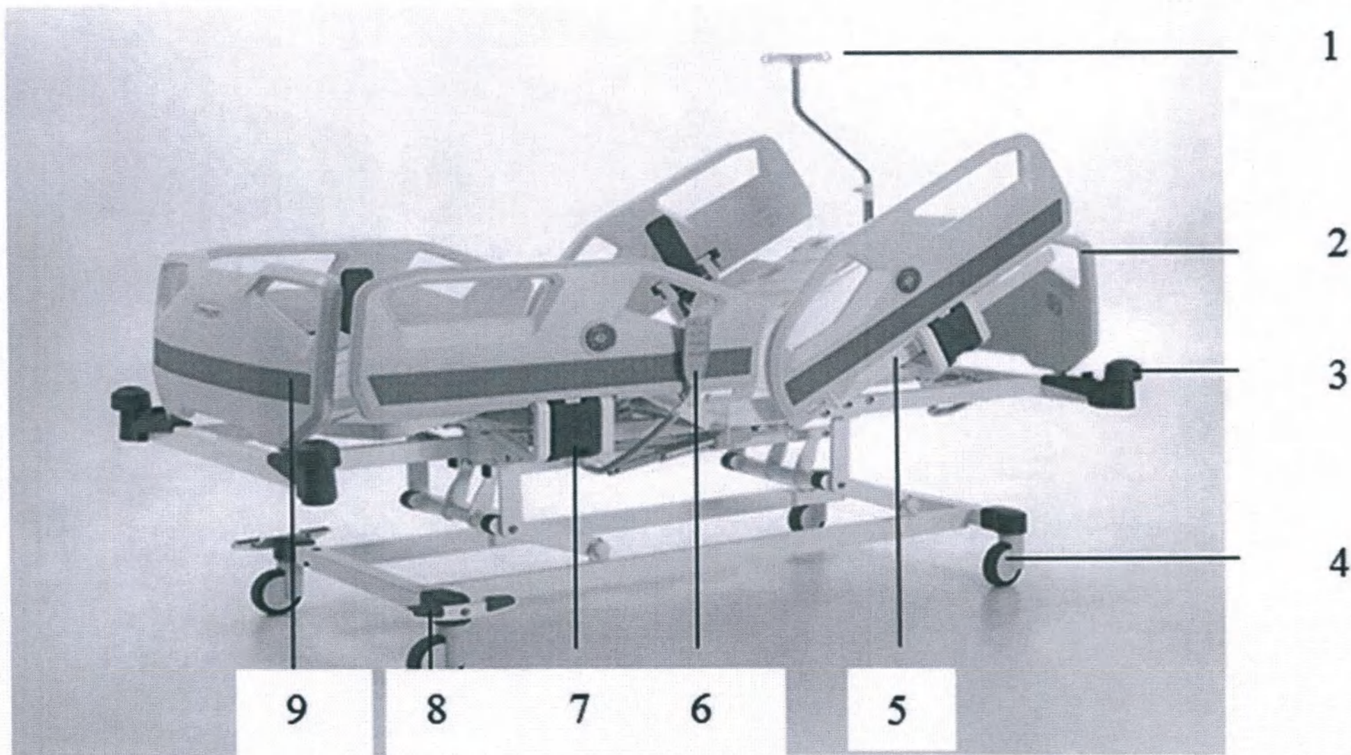
1. Стойка инфузионная; 2. Панель изголовья; 3. Бампер защитный; 4. Колесо Ø125мм; 5. Ограждение боковое; 6. Пульт управления ручной; 7. Механизм открытия/закрытия бокового ограждения; 8. Система блокировки колёс; 9. Панель изножья
