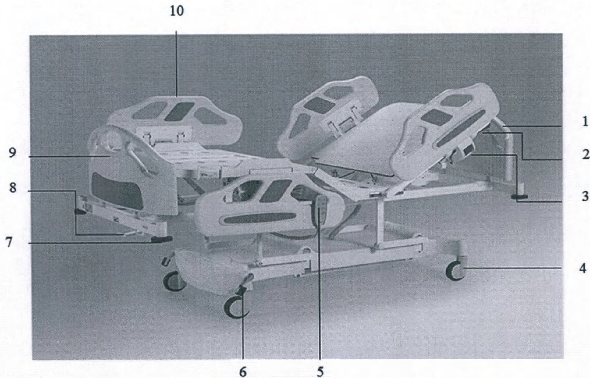
1. Панель изголовья съёмная. 2. Рычаг CPR. 3. Механизм открытия/закрытия бокового ограждения. 4. Колеса Ø125 мм. 5. Пульт управления ручной. 6. Система блокировки колес. 7. Бампер защитный. 8. Регулировка положения Тренделенбурга. 9. Панель изножья. 10. Ограждение боковое
