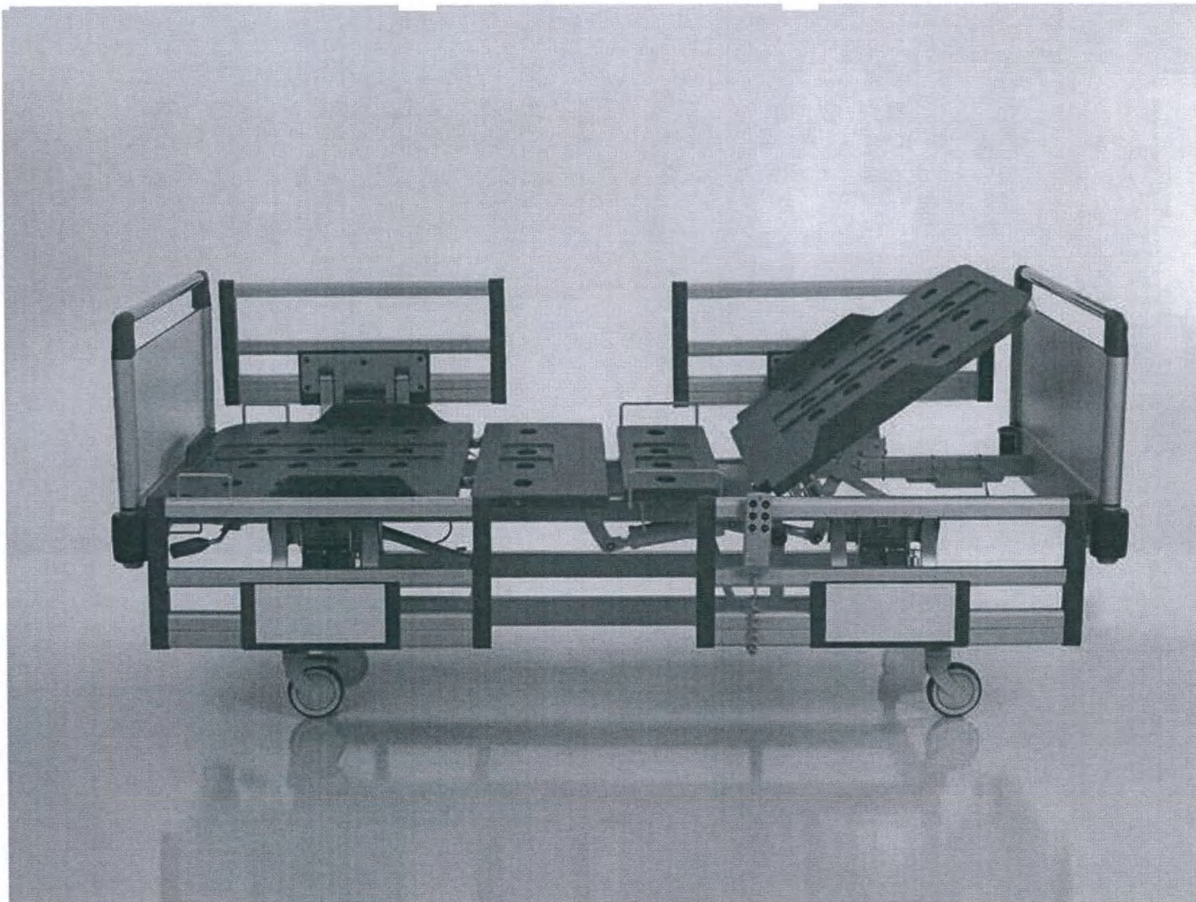
Вариант исполнения: кровать медицинская электрическая NITROCARE с принадлежностями серия Compact NITRO HB 2110
