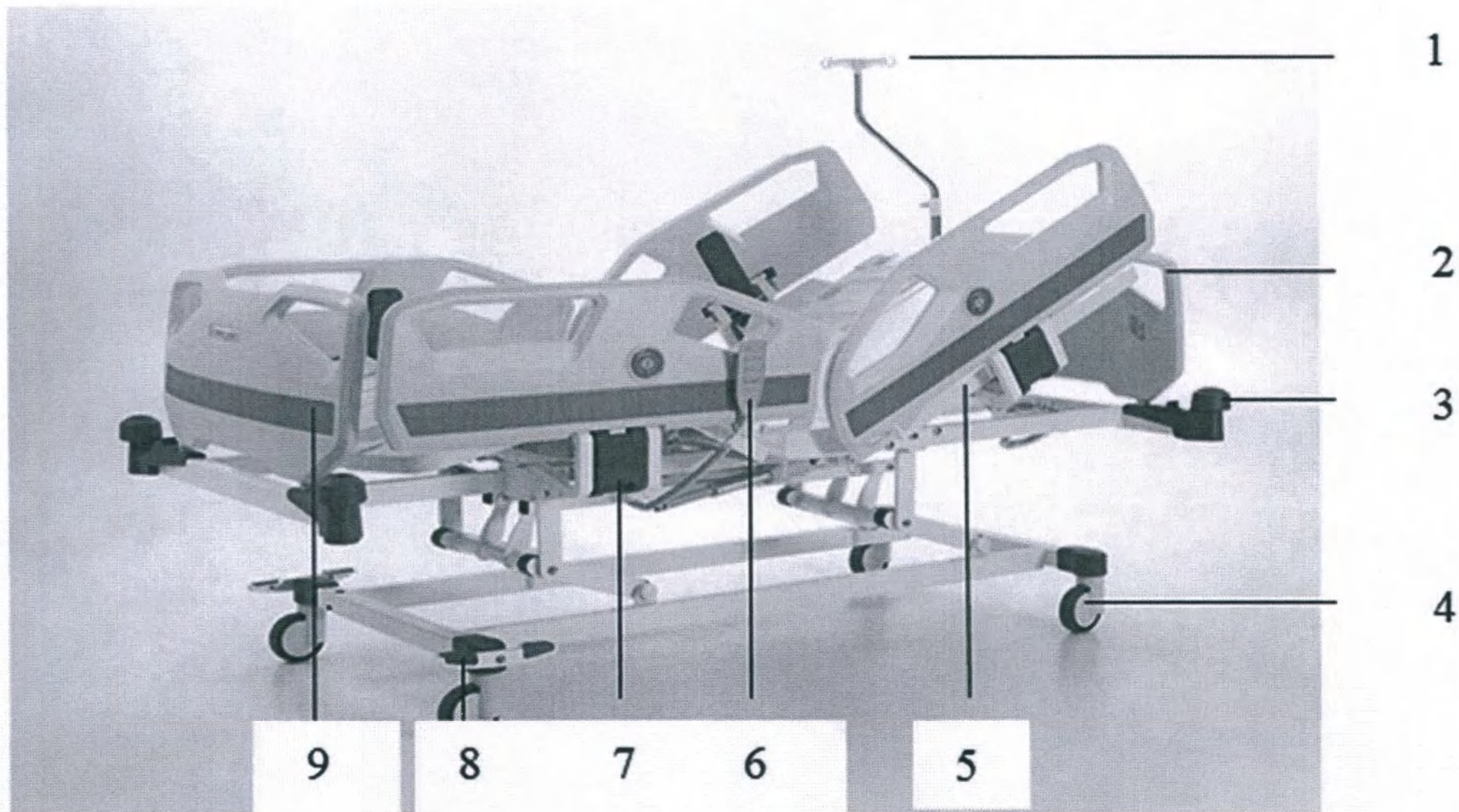
1. Стойка инфузионная. 2. Панель изголовья. 3. Бампер защитный. 4. Колесо Ø125мм . 5. Ограждение боковое. 6. Пульт управления ручной. 7. Механизм открытия/закрытия бокового ограждения. 8. Система блокировки колёс. 9. Панель изножья
