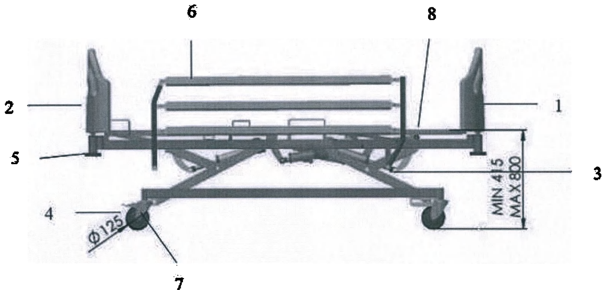
1. Панель изголовья. 2. Панель изножья. 3. Механизм открытия/закрытия бокового ограждения (система блокировки). 4. Колесо \Phi 125 мм. 5. Бампер защитный. 6. Ограждение боковое. 7. Педаль тормоза. 8. Поверхность ложа
