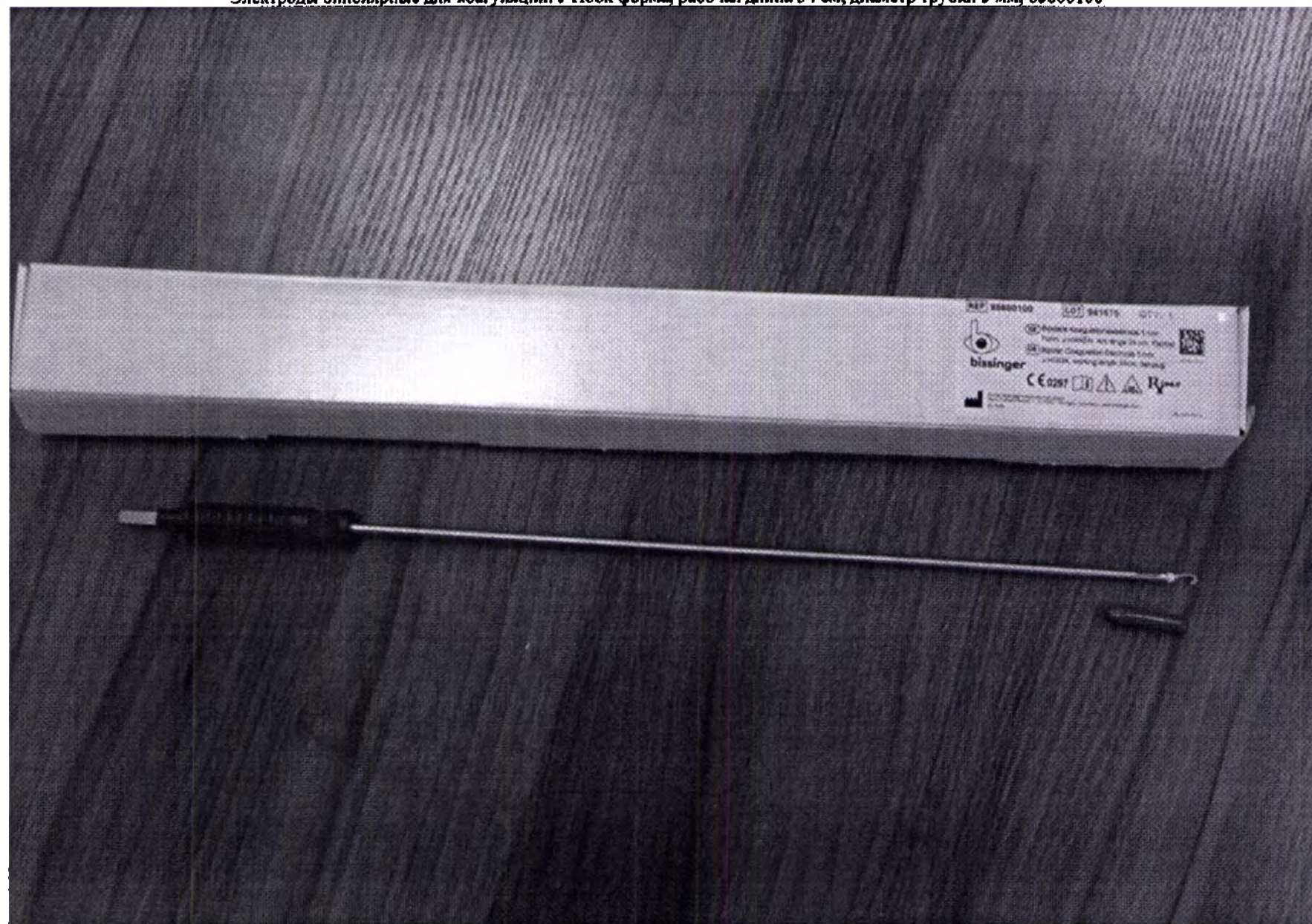
Электроды биполярные для коагуляции: J-Hook форма, рабочая длина 34 см, диаметр трубки 5 мм, 85600100
