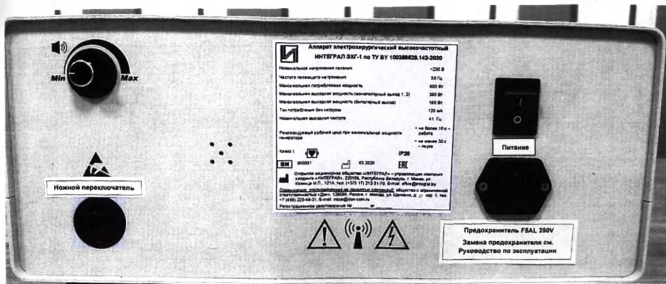
Фотографическое изображение аппарата электрохирургического высокочастотного ИНТЕГРАЛ ЭХГ-1 (генератор электрохирургический) – вид сзади.
