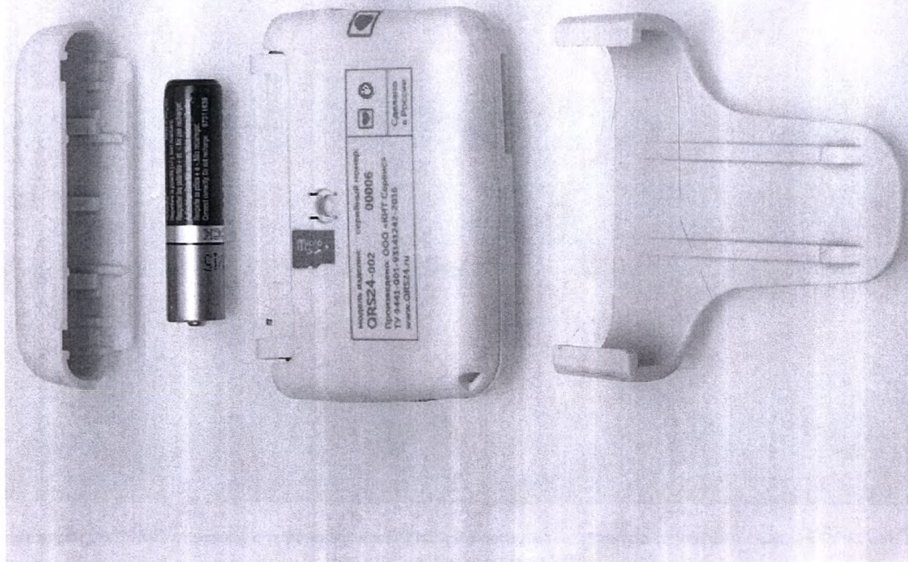
Регистратор QRS24-002 с Клипсой для крепления комплекса на поясе пациента и Элементом питания (AAA)
