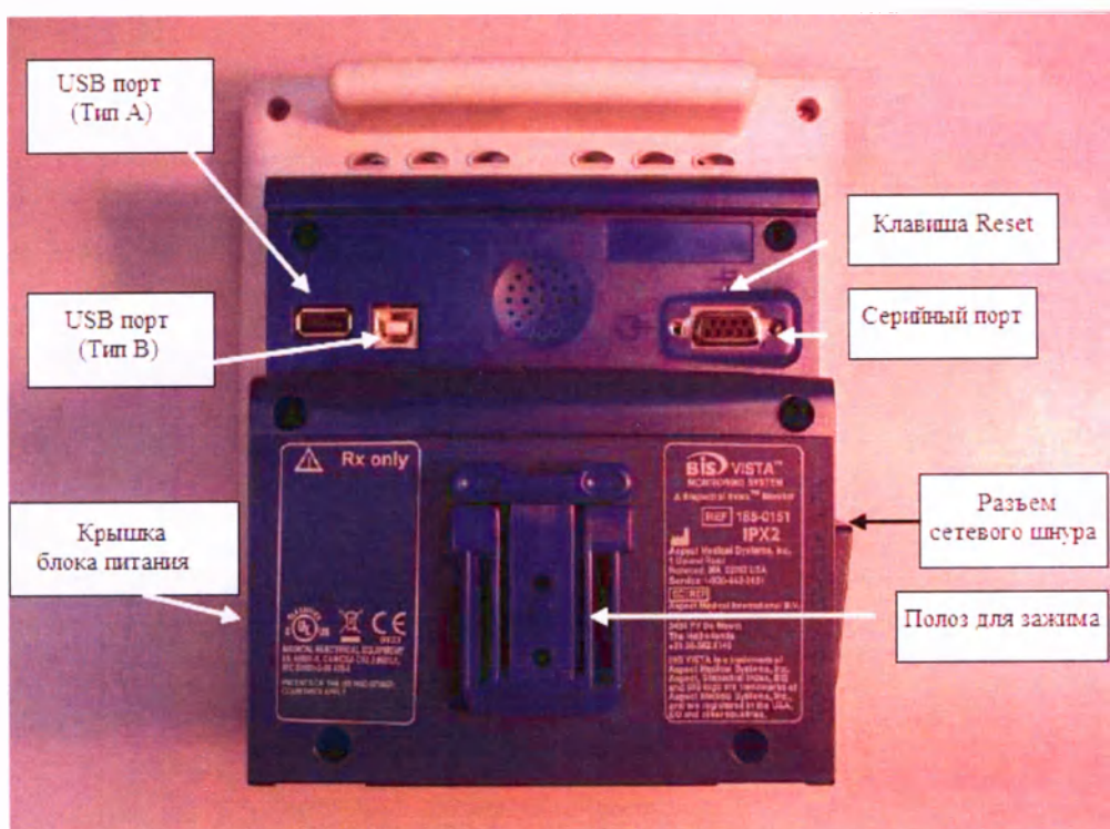
Задняя панель Основного блока BIS Vista
