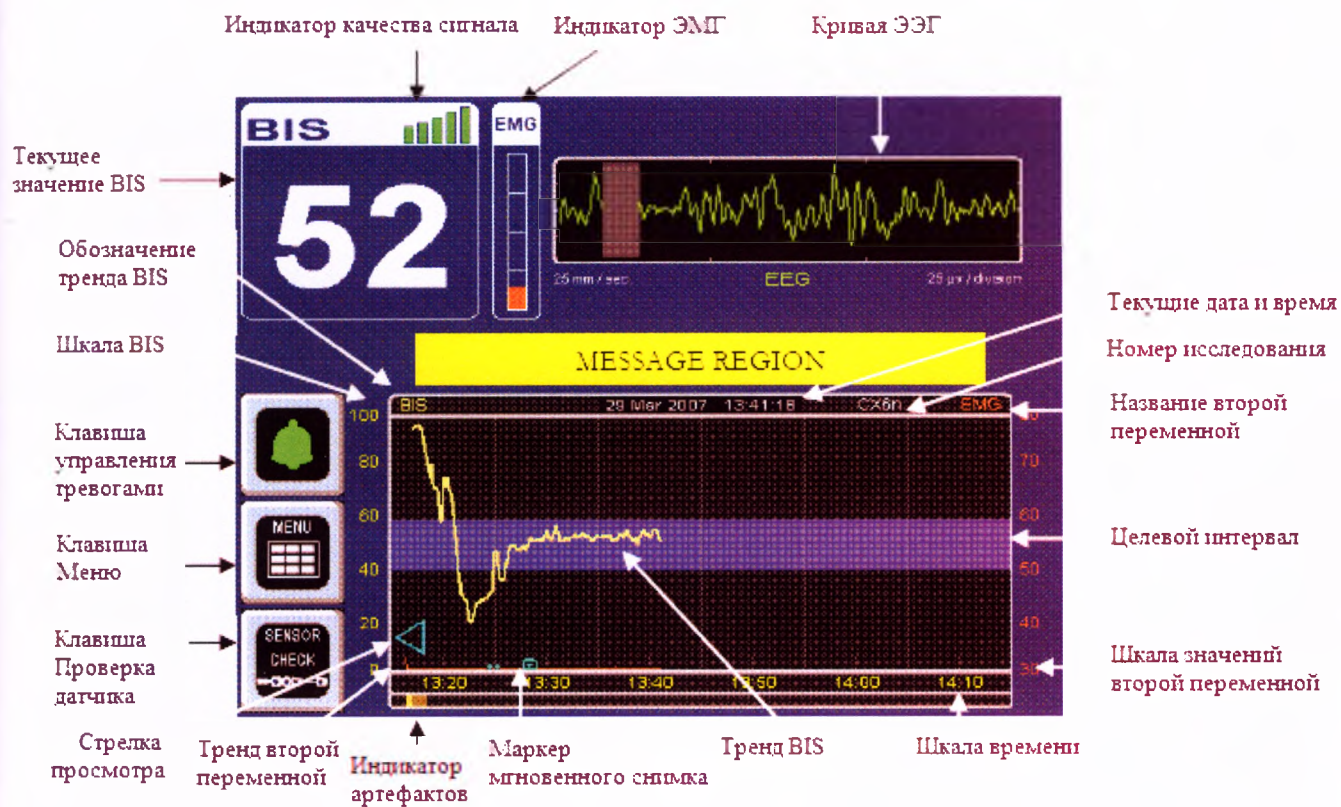
Панель дисплея Основного блока
