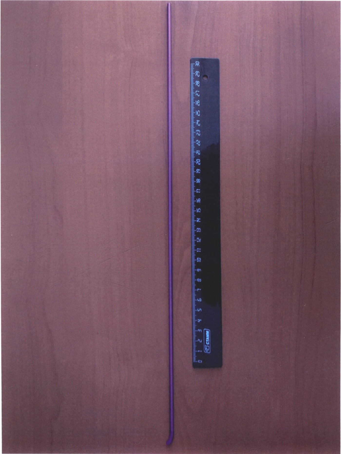
Штифт ТЕН гибкий титановый, Ø 4.0 мм, длина 440 мм. Общий вид.
