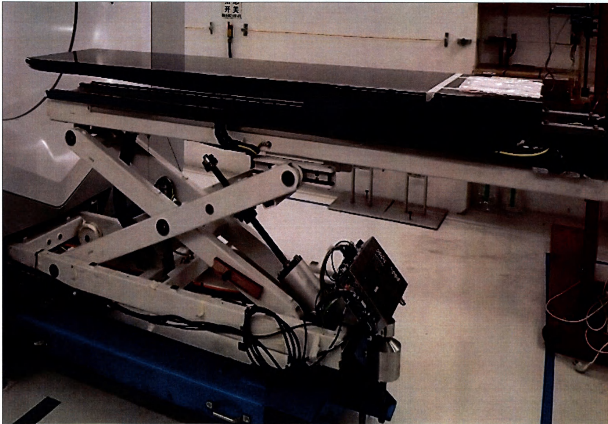
96. Стол пациента.
