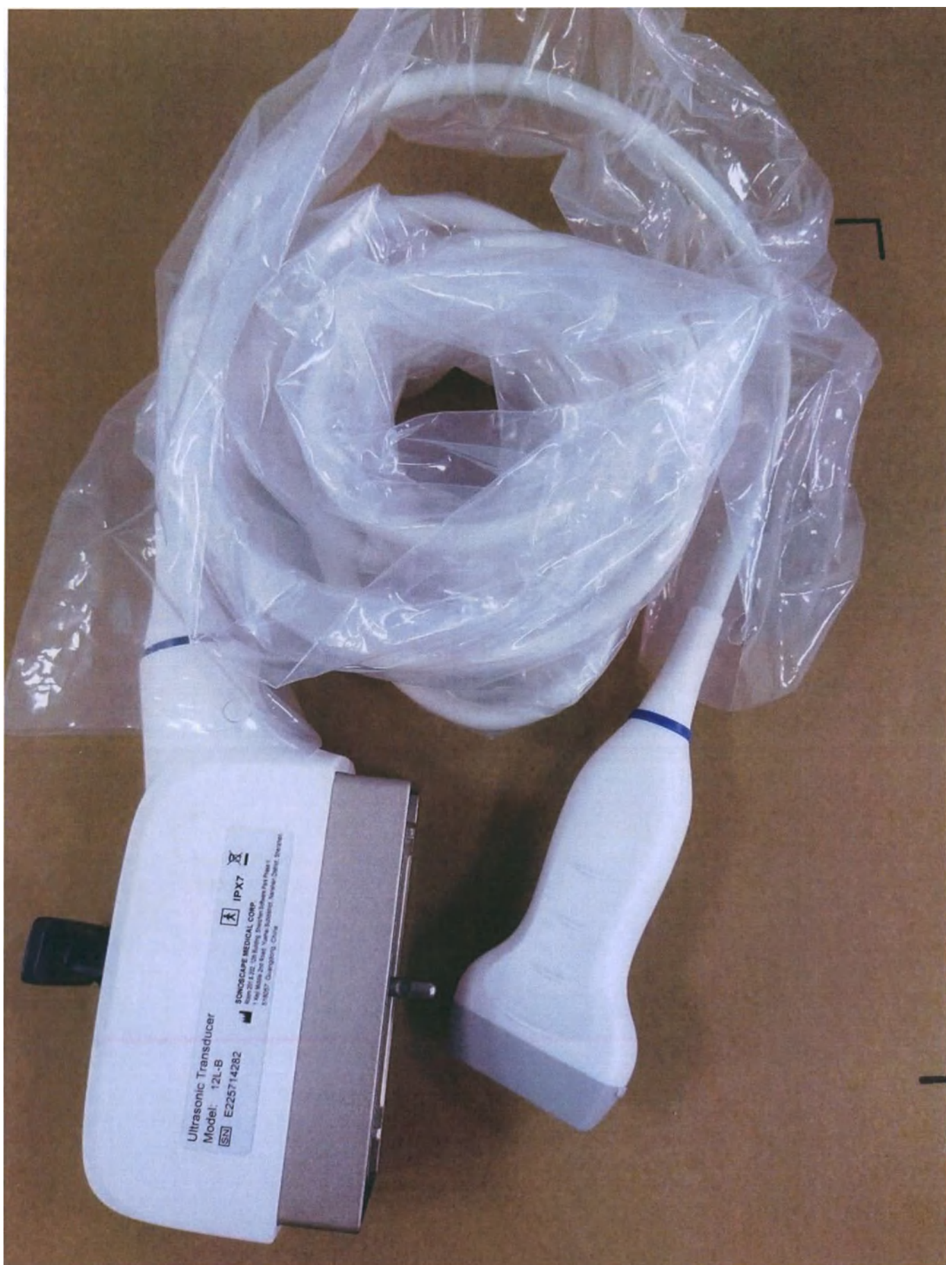
25. Датчик линейный ультразвуковой 12L-B
