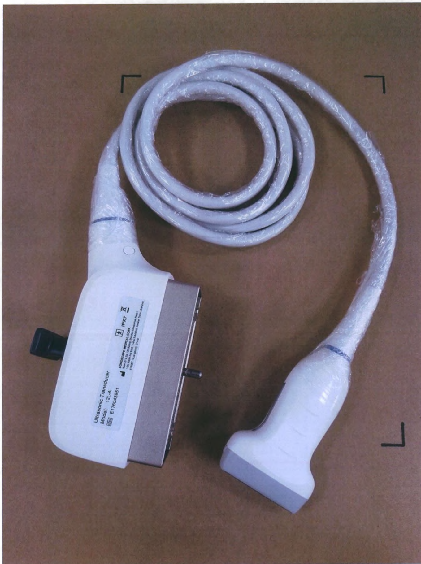
24. Датчик линейный ультразвуковой 12L-A
