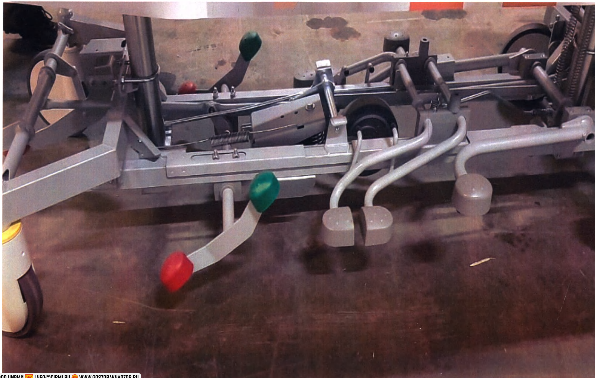
1.9. Педальная система регулировки высоты и наклона ложа с 6-ю педалями интегрированная в ходовую часть (1 шт.).
