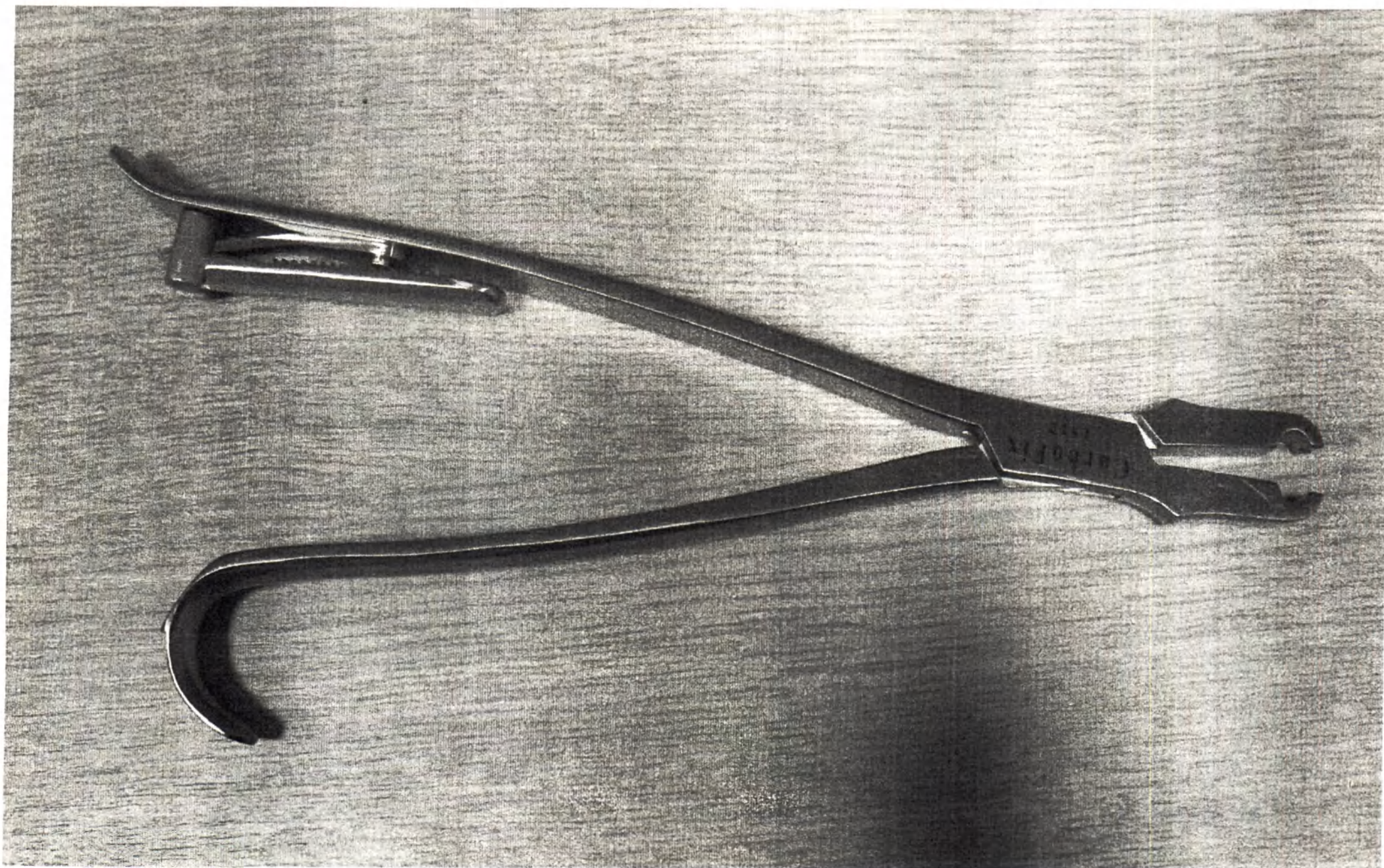
2.10. Держатель стержня
