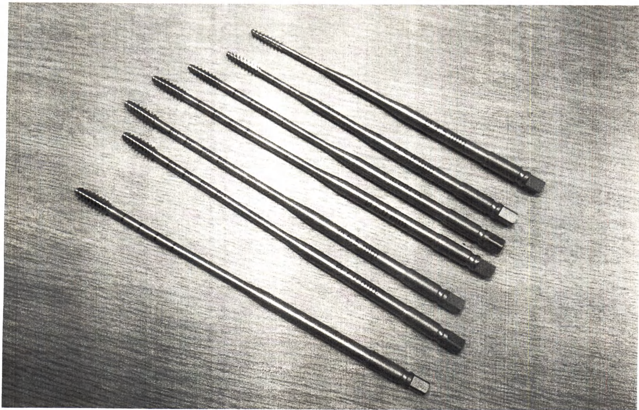
Метчик, Ø, мм: 4.5, 5.0, 5.5, 6.0, 6.5, 7.0, 7.5
