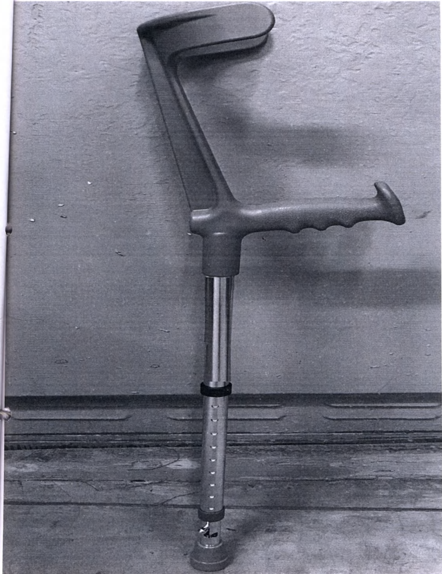
Рис.8 – Средства для реабилитации: костыль с опорой под локоть с УПС, модель Т.Р220У по ТУ 32.50.22-002-34380083-2018
