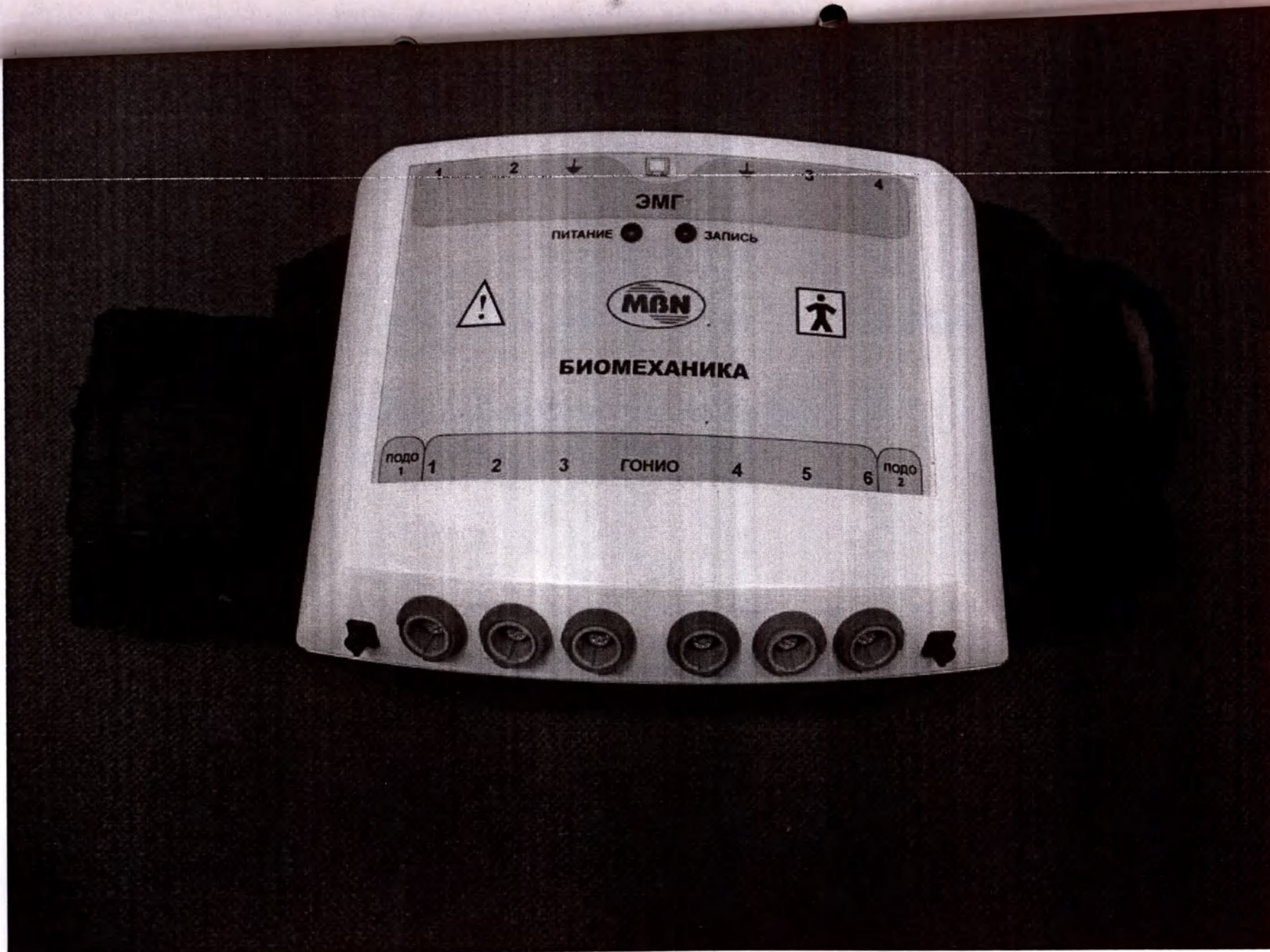
Фото 12 – Системный блок с поясом крепления
