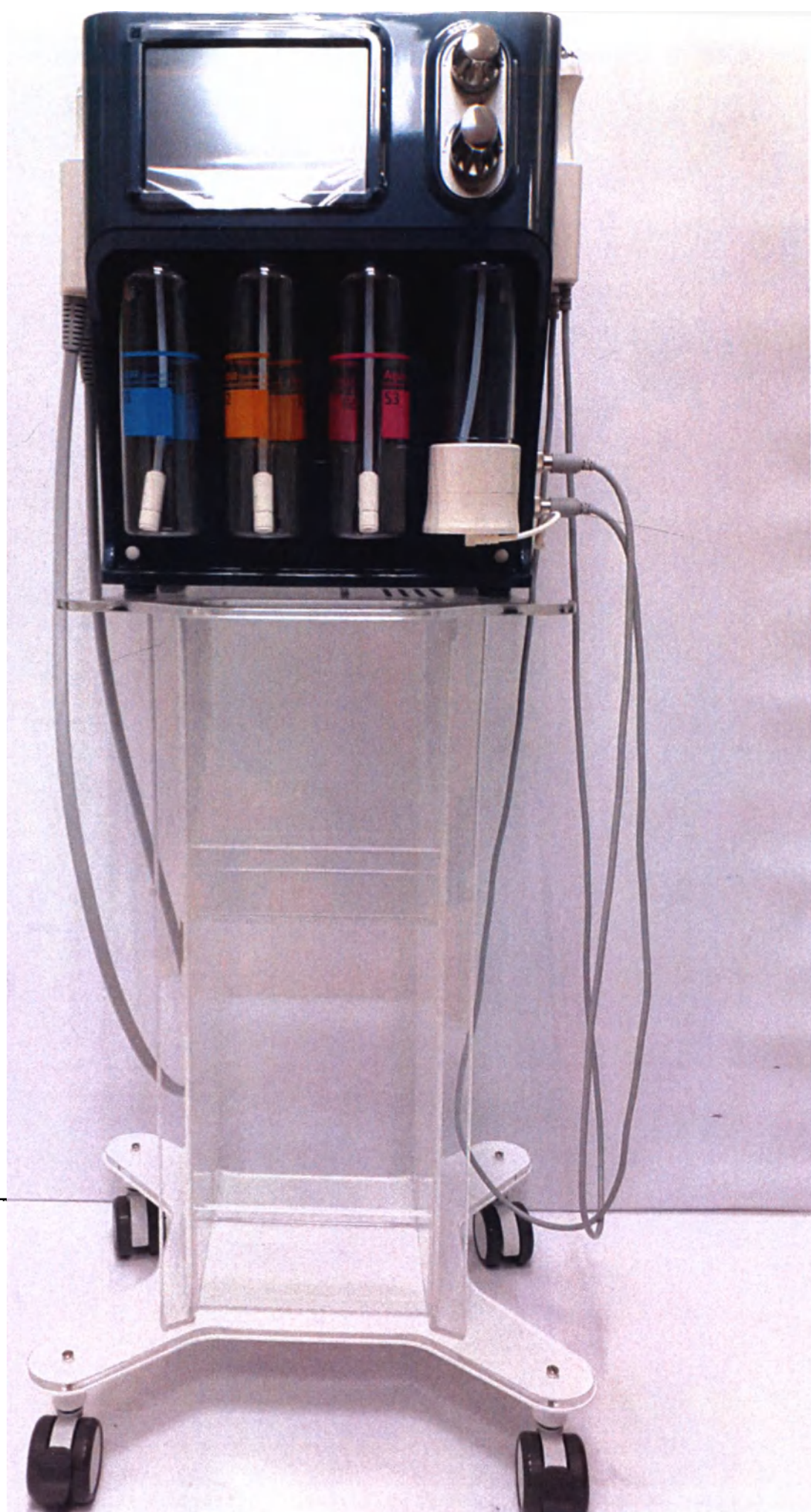
Фотографическое изображение 5. Аппарат косметологический Hydra с принадлежностями, в варианте исполнения: Hydra Touch H2, Hydra Beauty. Вариант исполнения Hydra Touch H2 - вид спереди. Аппарат установлен на тележку
