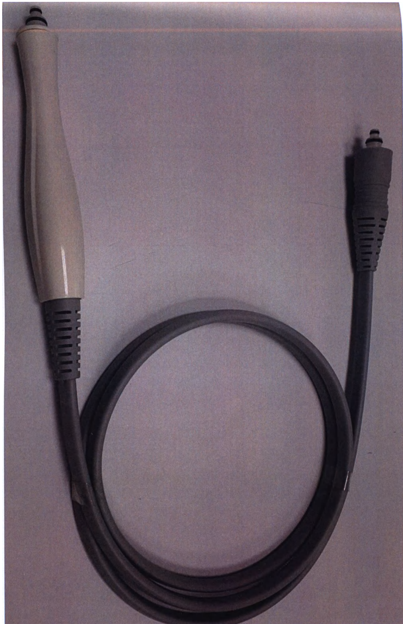
Фотографическое изображение 22. Аппарат косметологический Hydra с принадлежностями, в вариантах исполнения: Hydra Touch H2, Hydra Beauty. Вариант исполнения Hydra Beauty – Аппликатор Aqua без насадки
