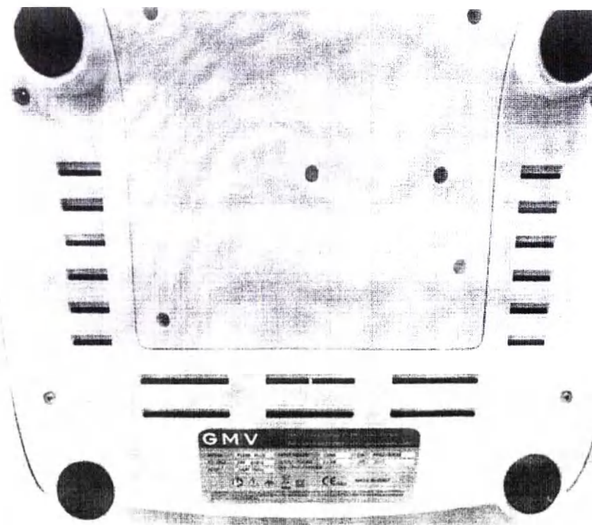
Фото 21. Вид нижней панели Plexr Plus с маркировочной табличкой.
