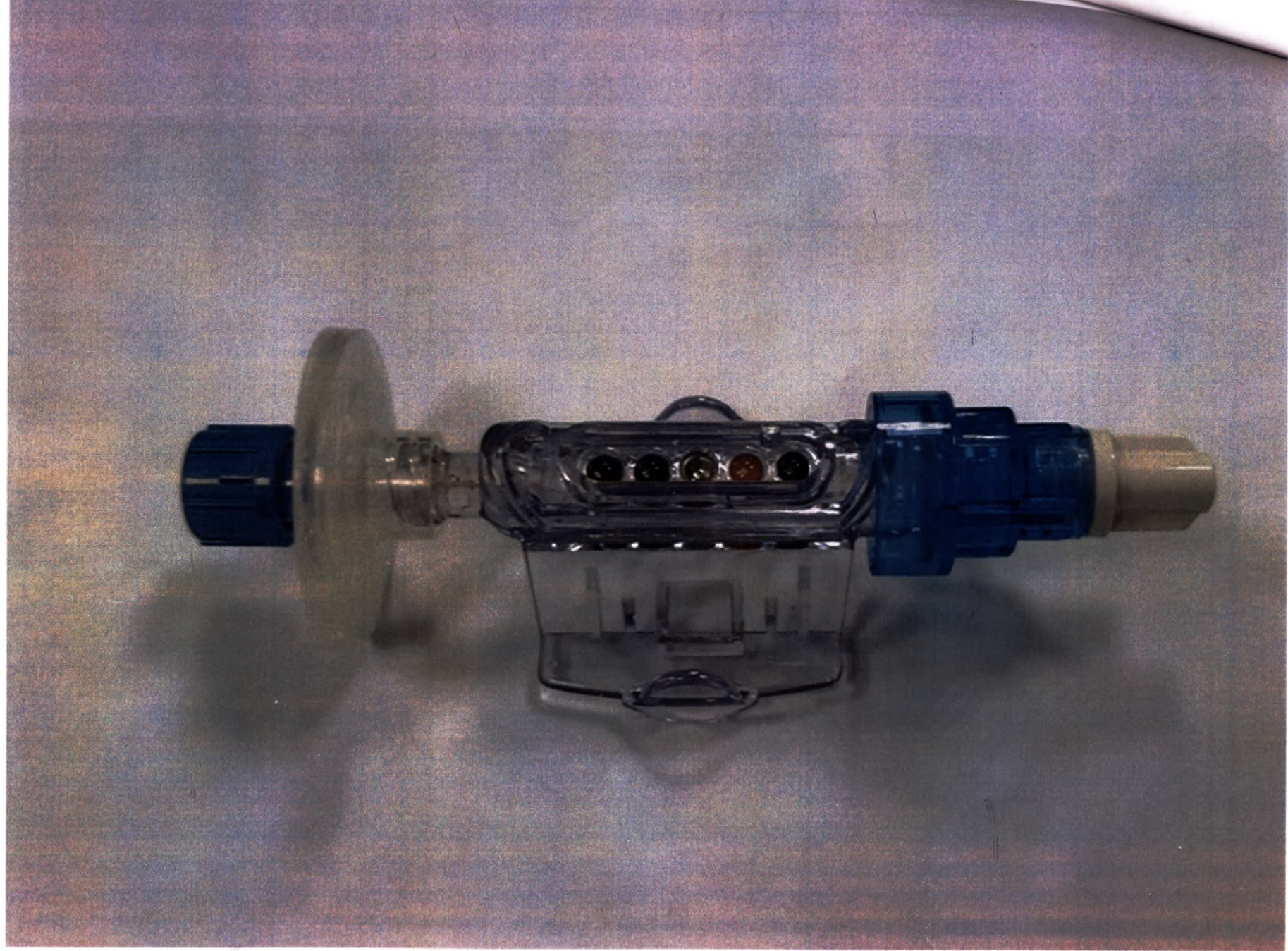
Датчик шунтирующий CDI с гепариновым покрытием, модель CDI510H, для системы мониторинга параметров крови CDI – внешний вид изделия
