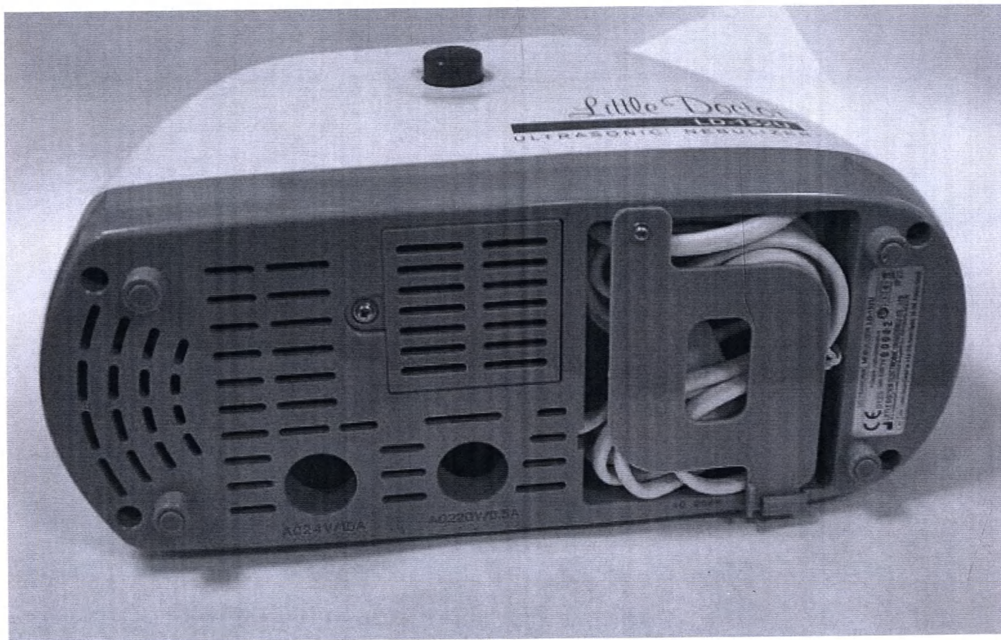
Ингалятор ультразвуковой LD-152U – основной блок, вид снизу.
