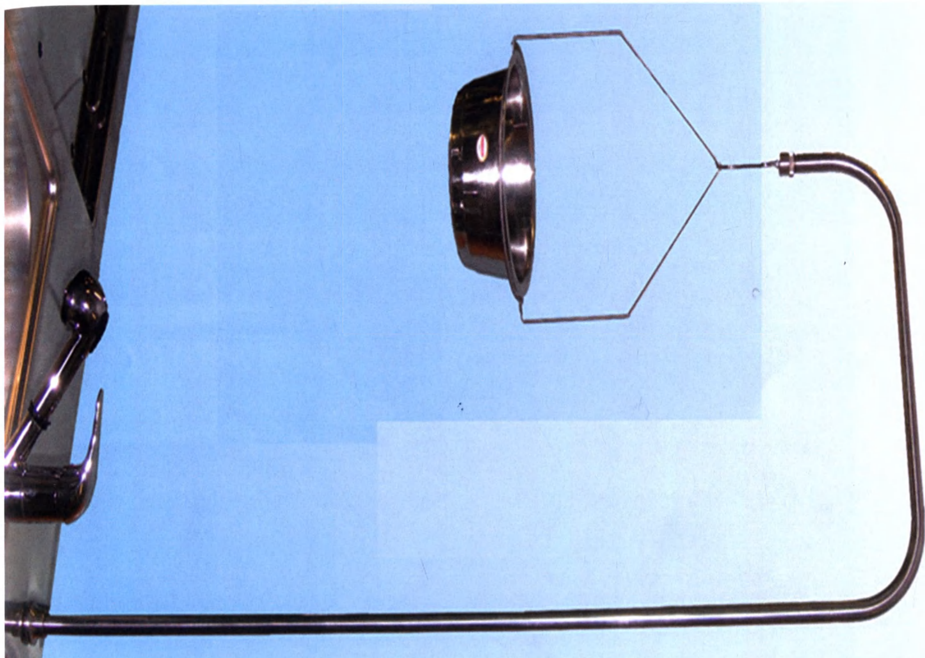
Стойка для весов ССВ-8С
