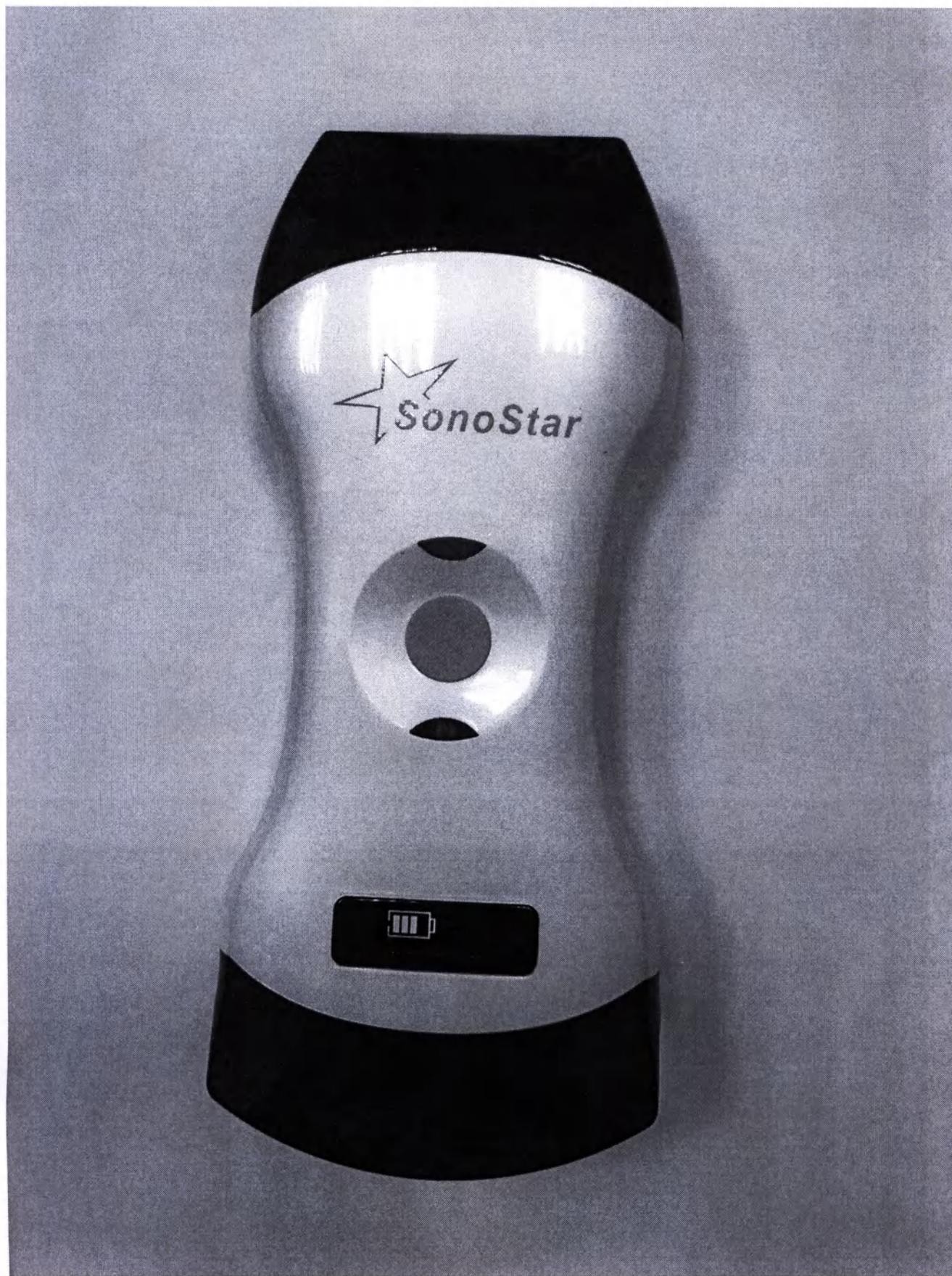
Сканер ультразвуковой беспроводного типа Uprobe-C5LC.
