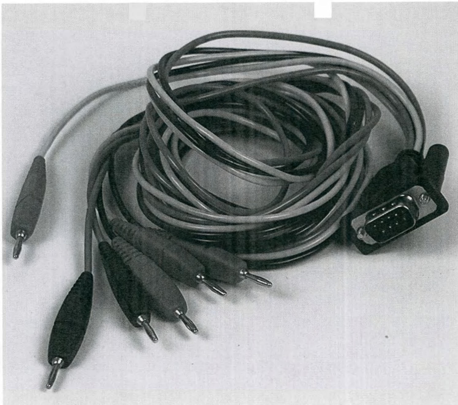
Аппарат электротерапевтический Neurodyn. Кабель пациента(1500 мм - разъем типа «банан» 2мм 2 шт.).
