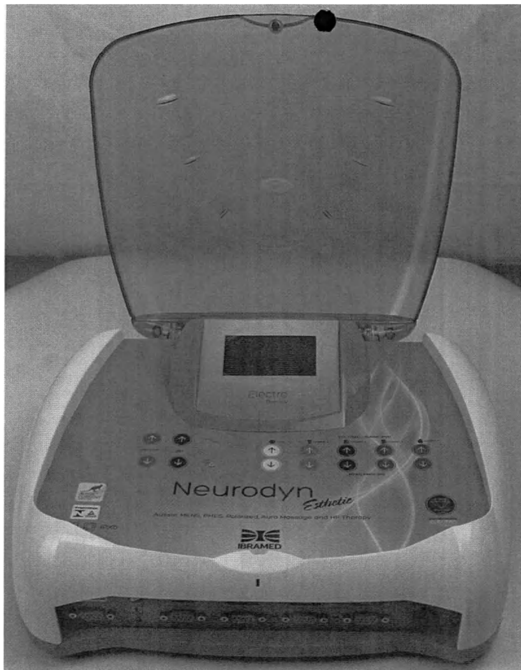
Аппарат электротерапевтический Neurodyn Esthetic. Основной блок.
