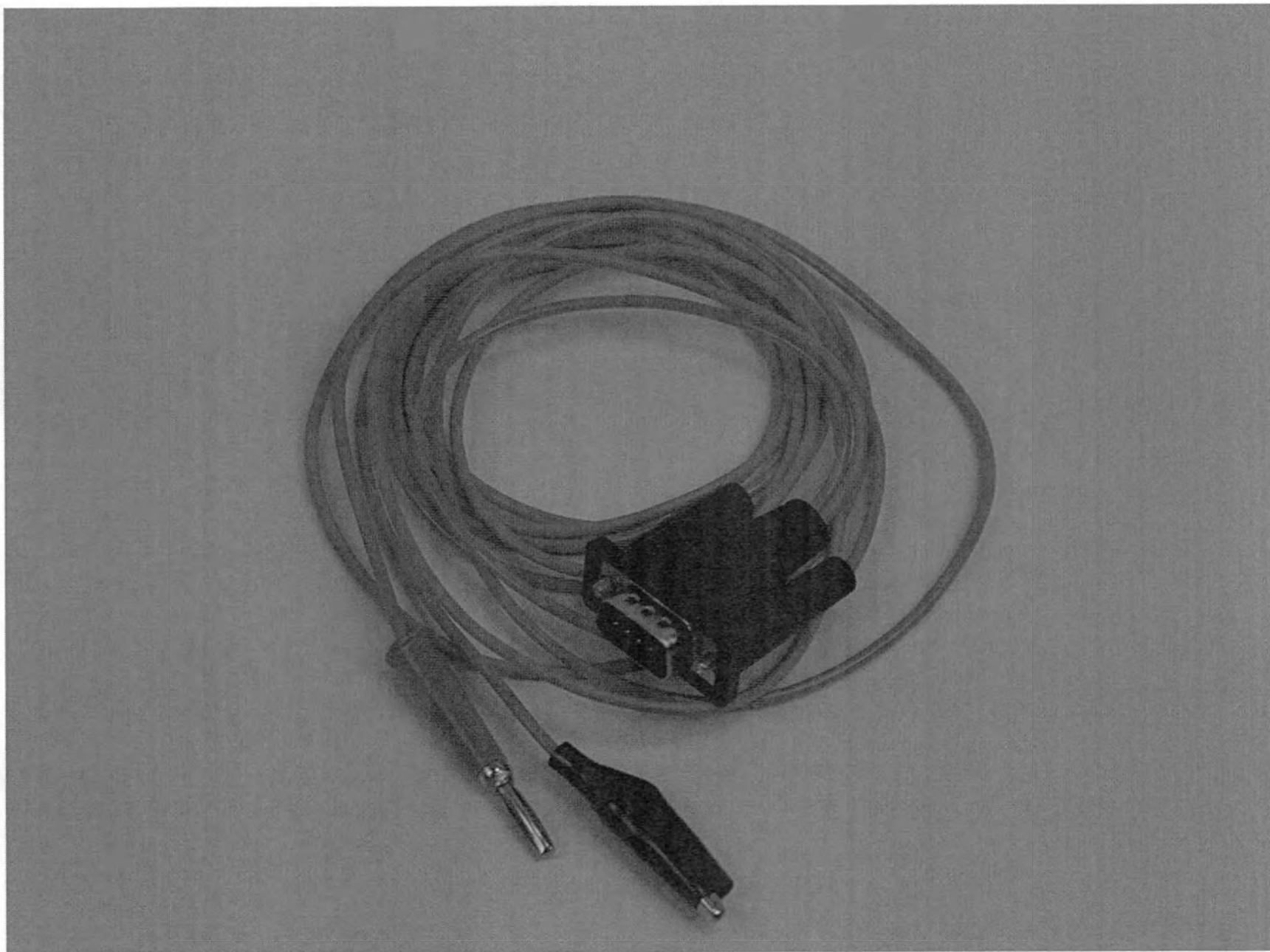
Аппарат электротерапевтический Neurodyn Esthetic. Кабель пациента (1500 мм - разъем типа «банан» 2 мм 1 шт., зажим типа «крокодил» несъемный 1 шт.).
