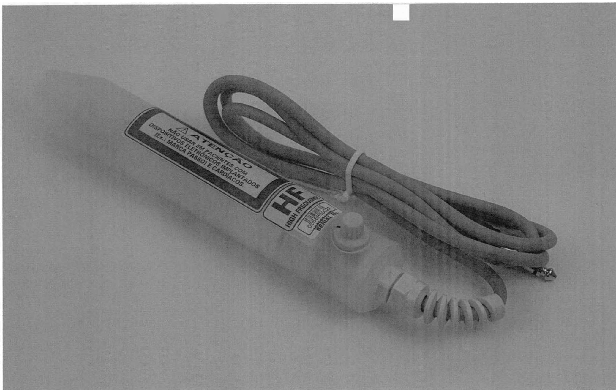
Аппарат электротерапевтический Neurodyn Esthetic. Ручка-электрод эстетическая для проведения электротерапии по лицу.
