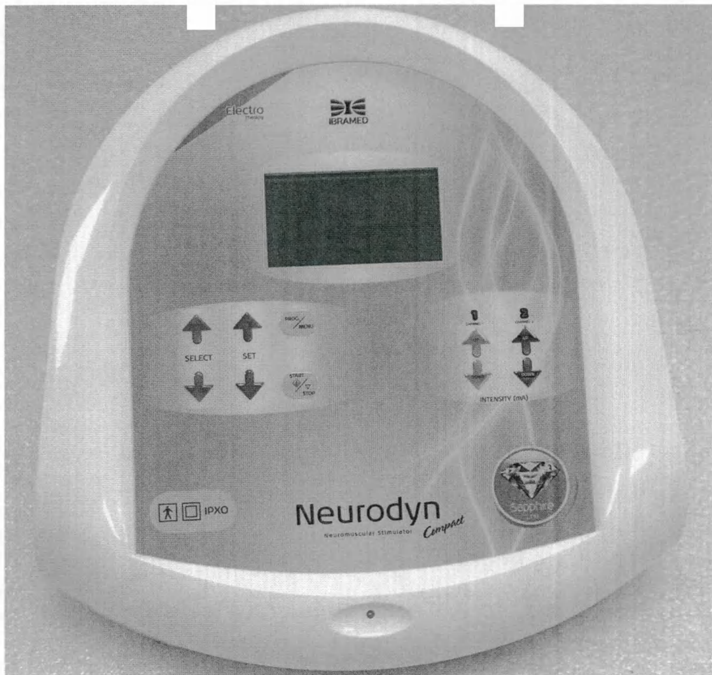
Аппарат электротерапевтический Neurodyn Compact. Основной блок.
