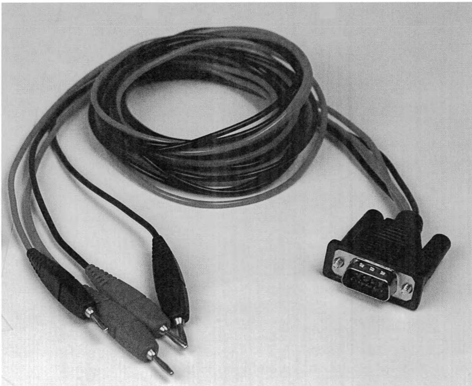
Аппарат электротерапевтический Neurodyn Compact. Кабель пациента (1500 мм - разъем типа «банан» 2мм).
