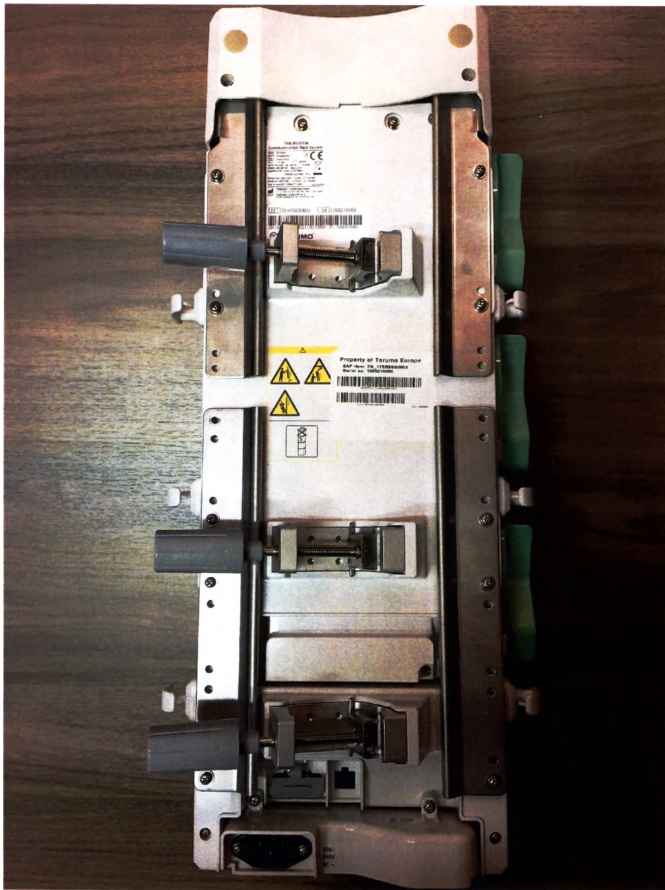
Стойка на примере: «Коммуникационная стойка TERUFUSION» (1)
