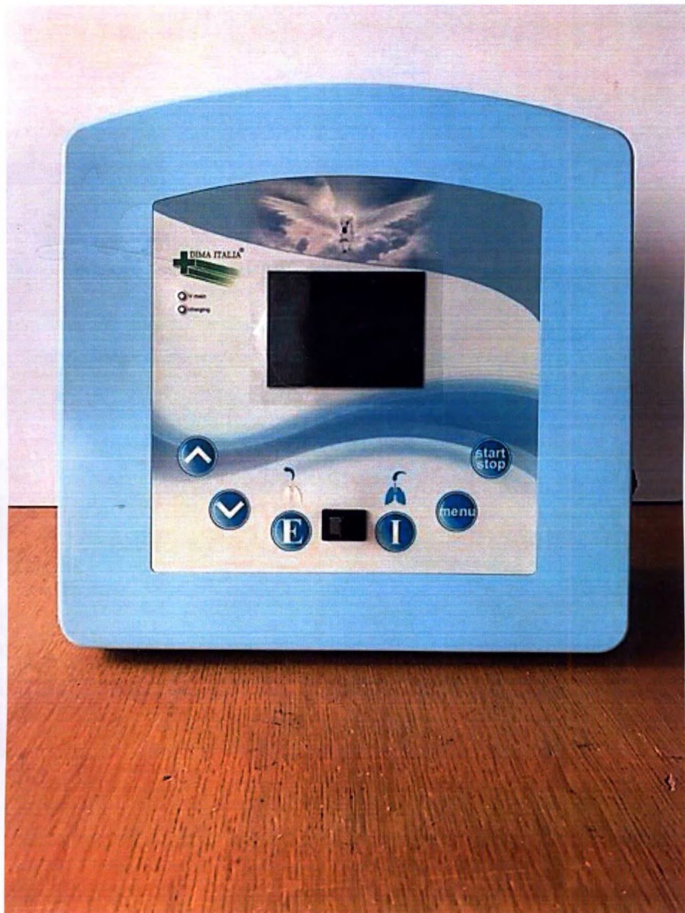
Блок основной (вентилятор), вариант исполнения: PEGASO PLUS Cough (вид спереди)
