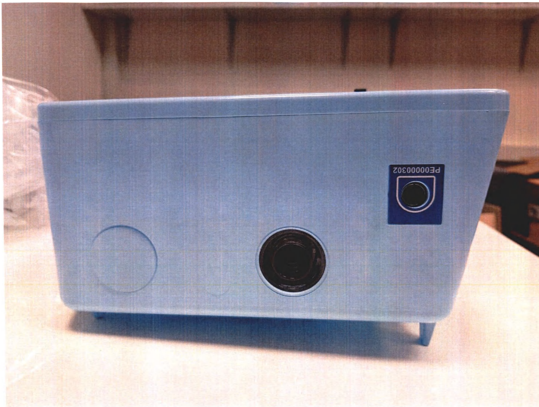
Блок основной (вентилятор), вариант исполнения: PEGASO PLUS Cough (вид слева)
