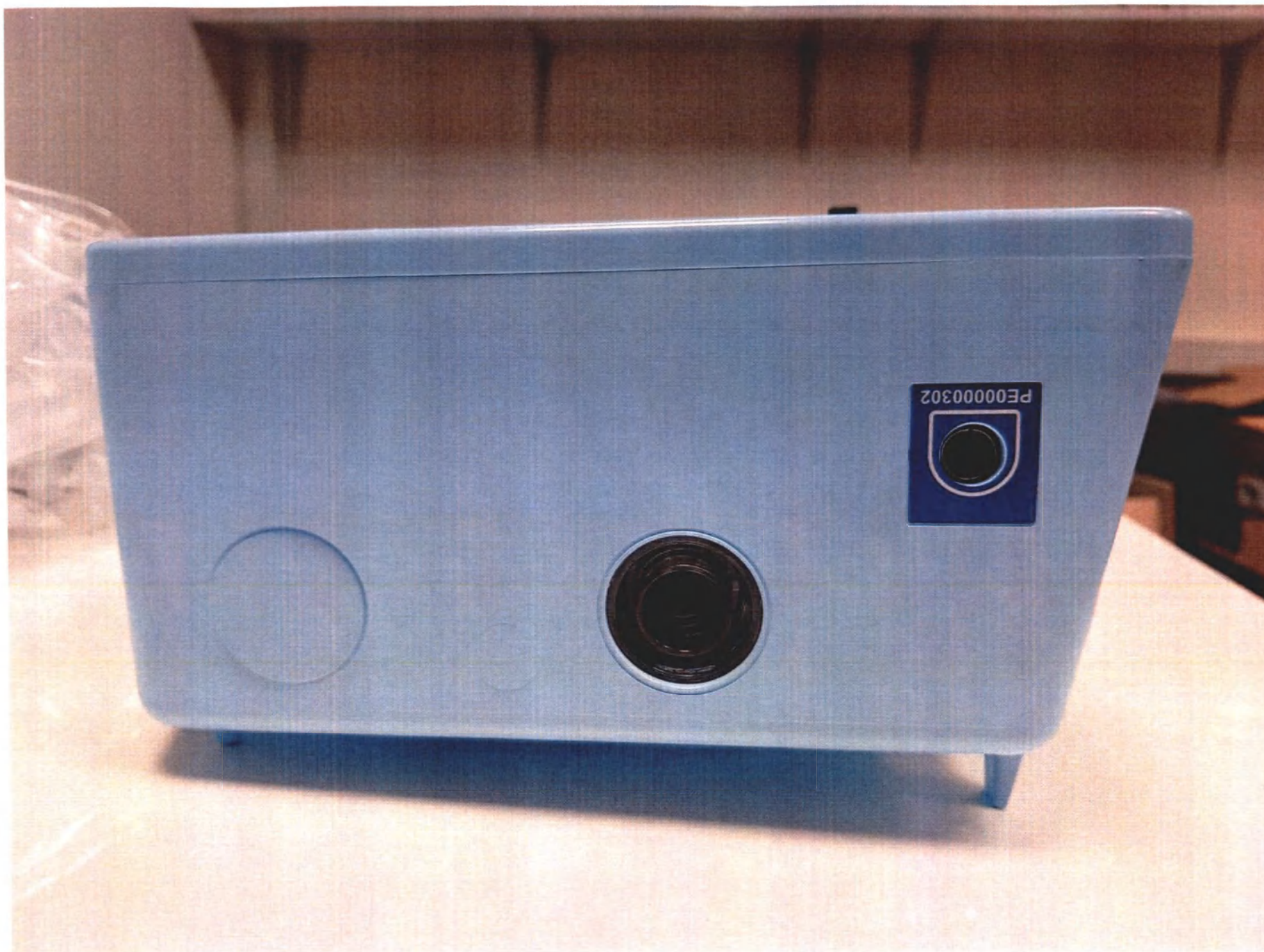
Блок основной (вентилятор), вариант исполнения: PEGASO PLUS Combi (вид слева)
