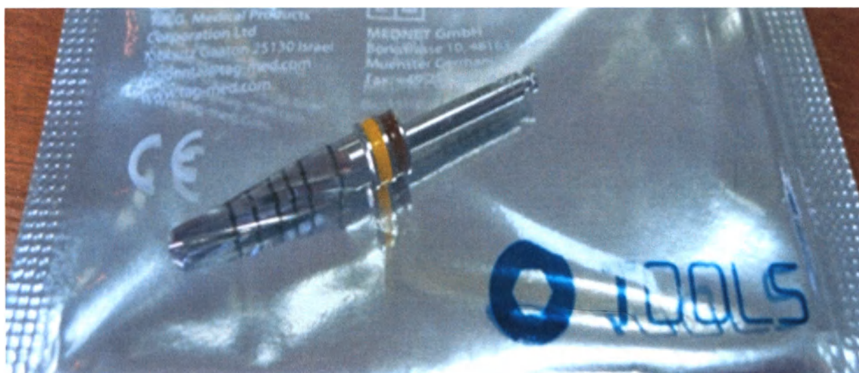
5.Фреза коническая
