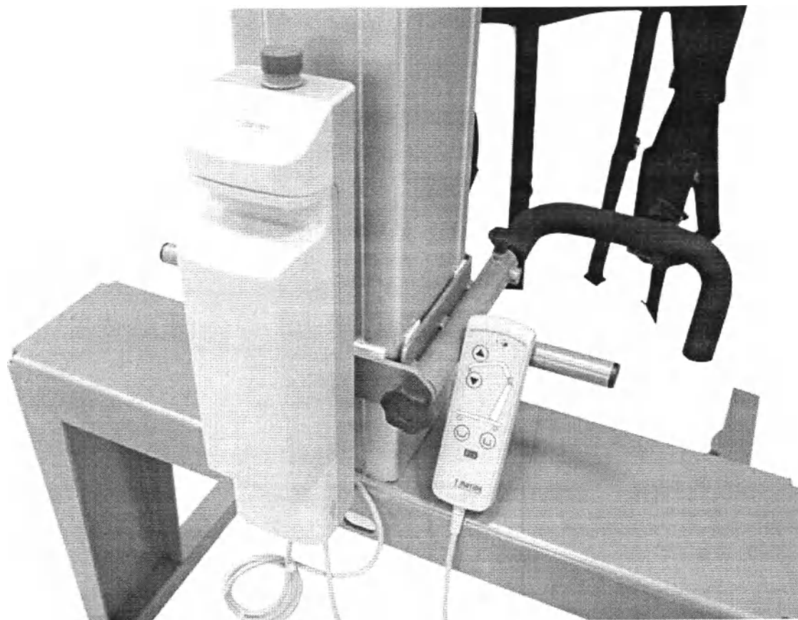
Дополнительный аккумулятор (емкость 5 А•ч)
