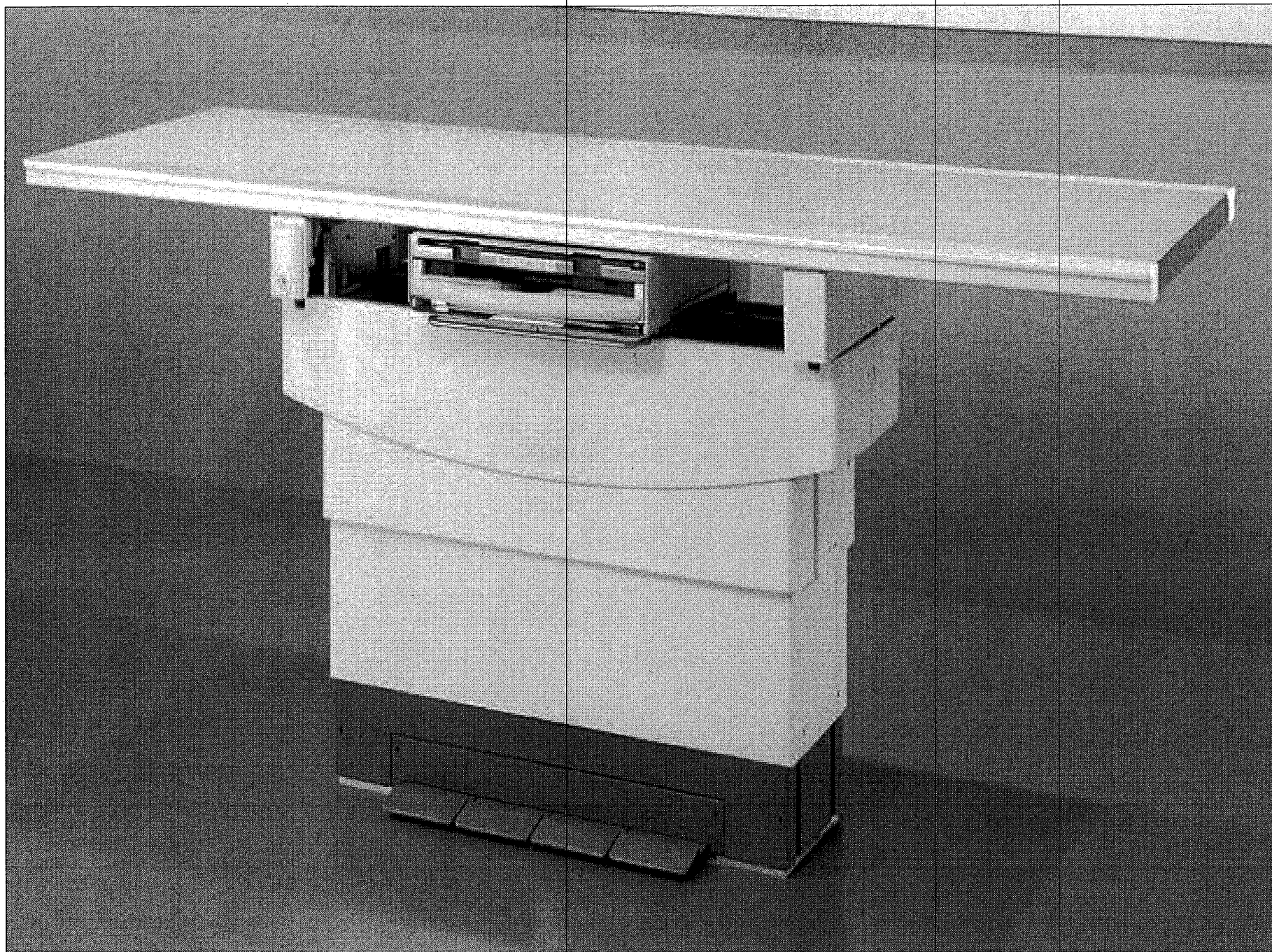
2.1 Столы для пациента (от 1 до 2 штук).
