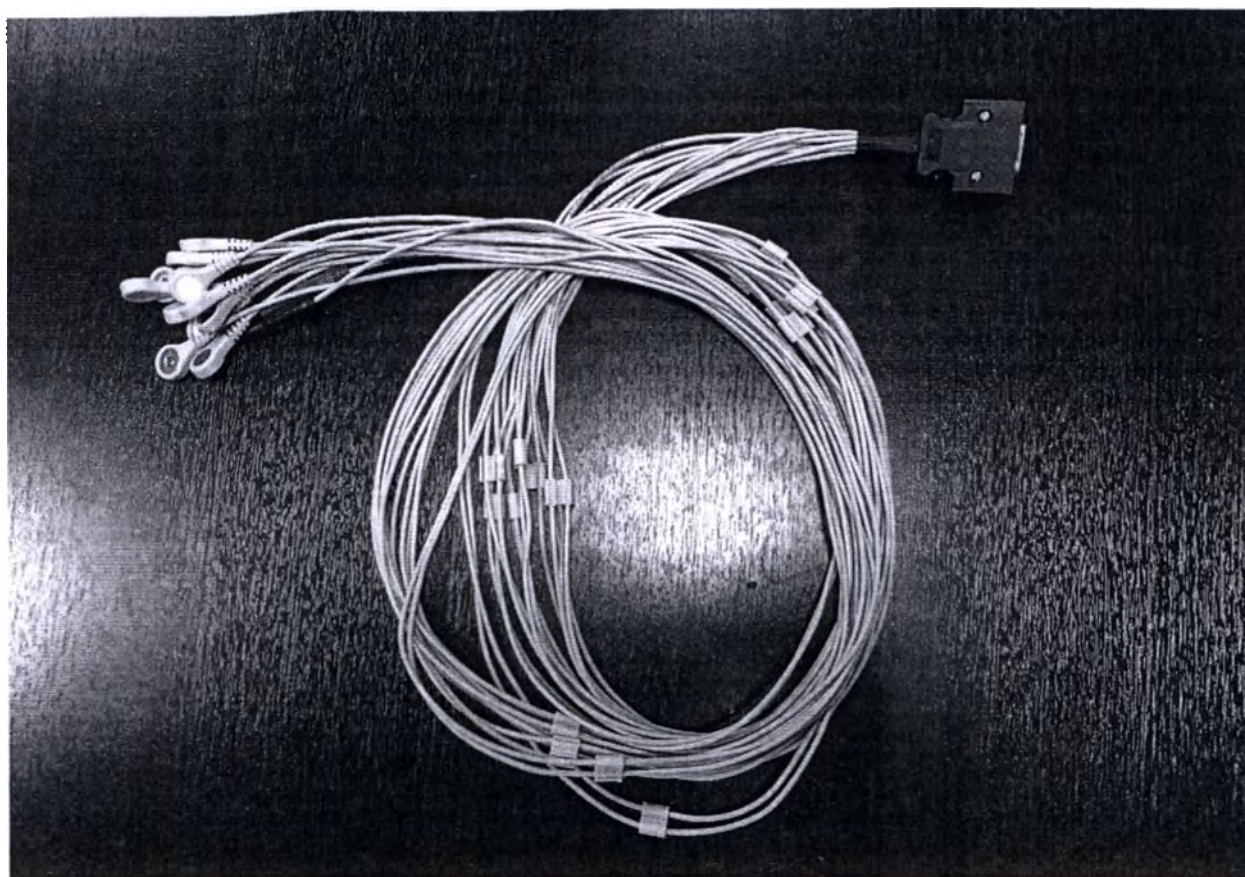
Биоэлектрический кабель MDR26 на примере Биоэлектрического кабеля MDR26 шестиканального
