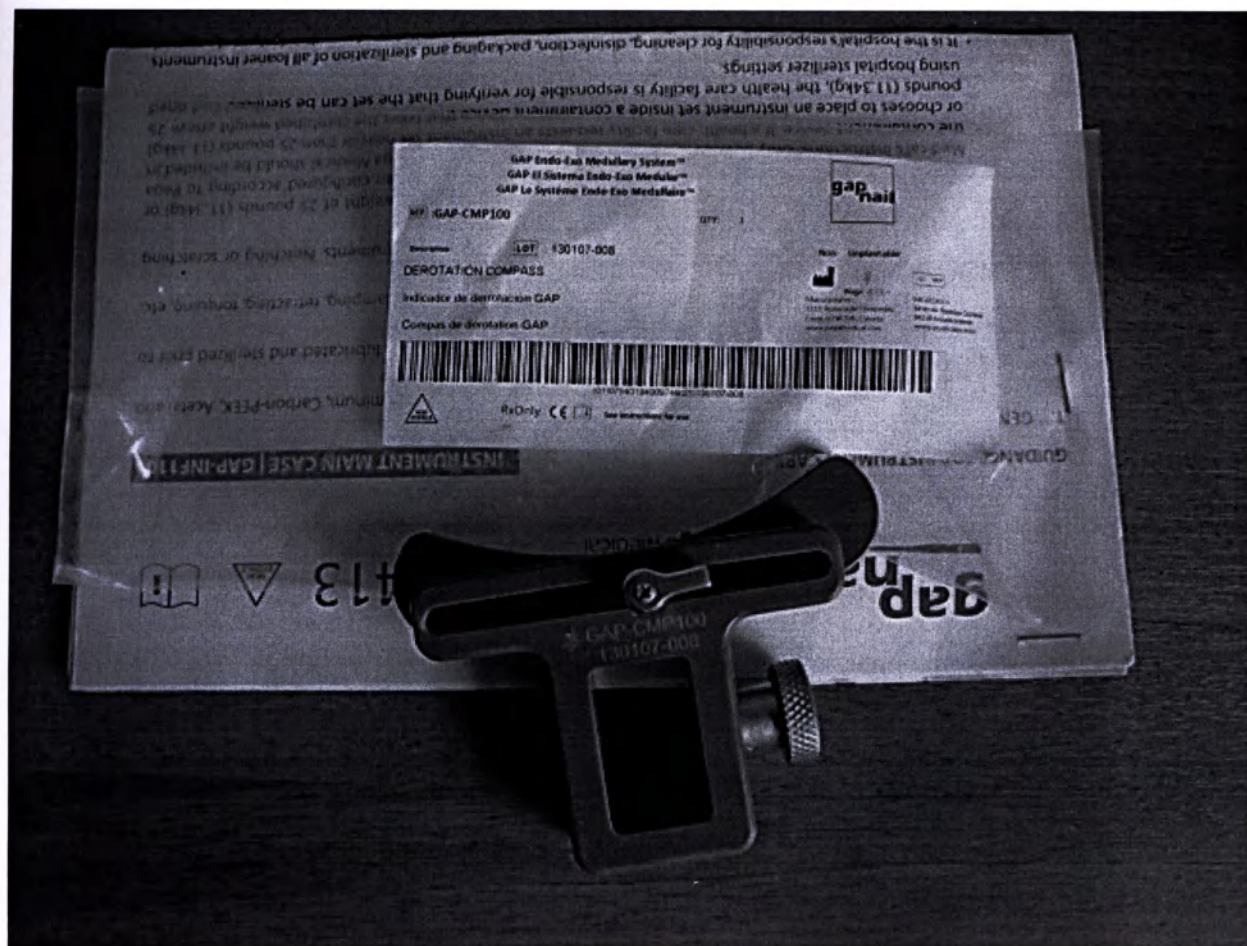
GAP-CMP100 Определитель ротации
