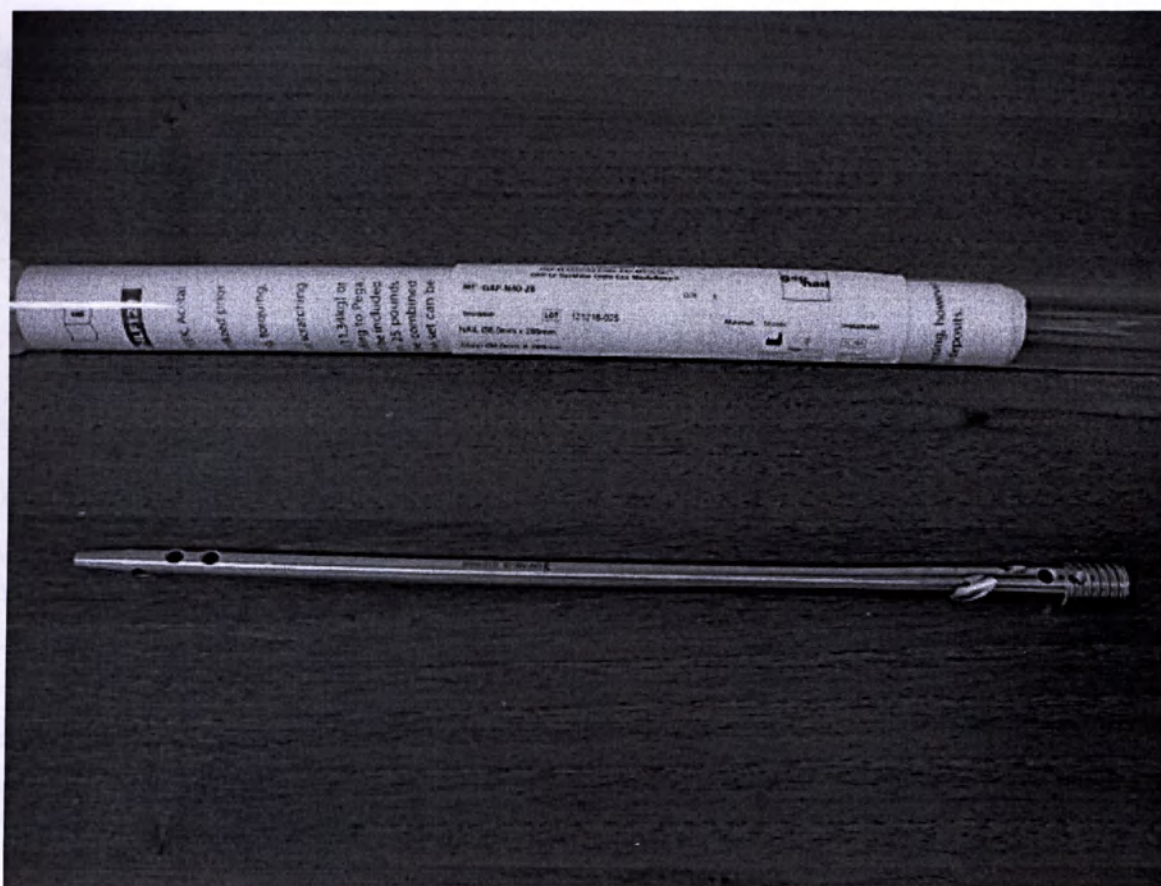
GAP-N80-28 Штифт GAP Nail, Ø 8,0 мм, длина 280 мм
