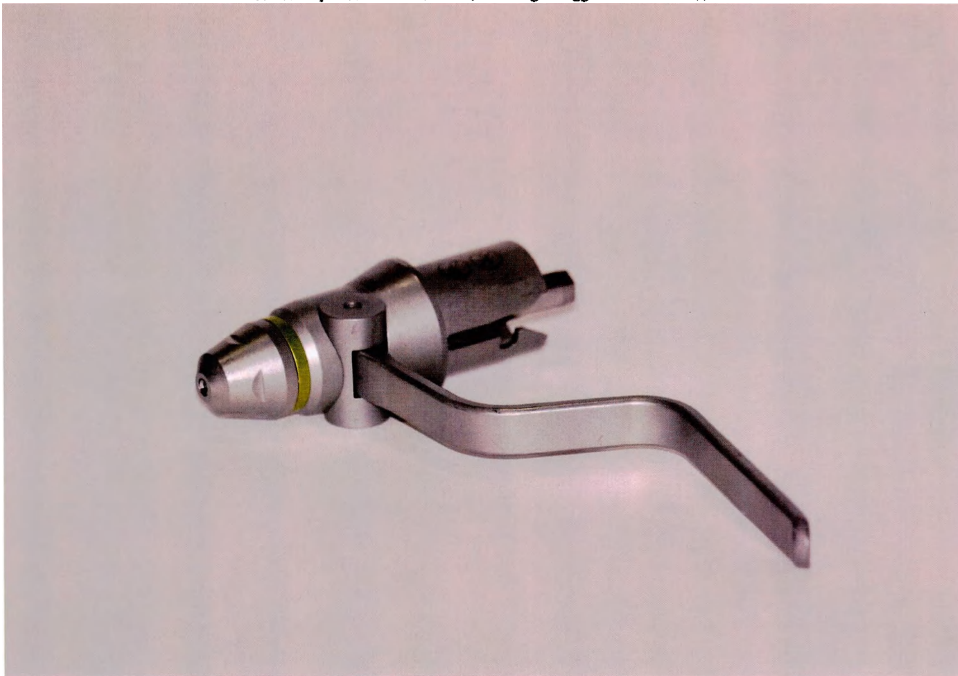
Насадка для проведения спиц PPE II, PPP Single Trigger Pin Driver. Изделие.
