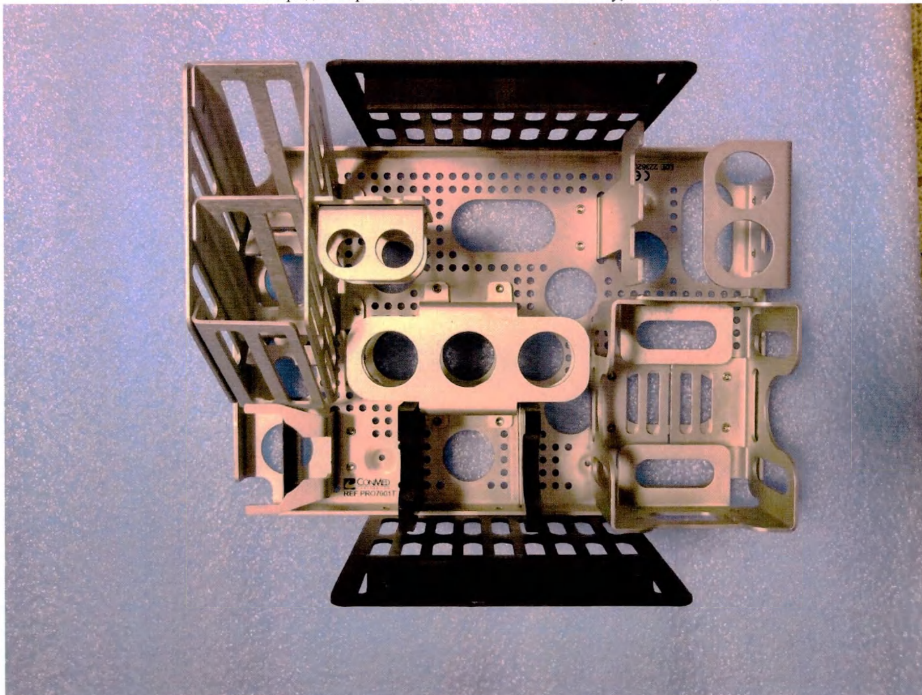
Лоток контейнера для стерилизации HALL 50 1/2-Size Inner Tray, Drill Set. Изделие.
