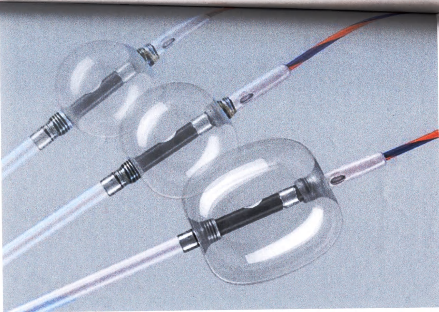
Катетер TXR-8.5-12-15-B
