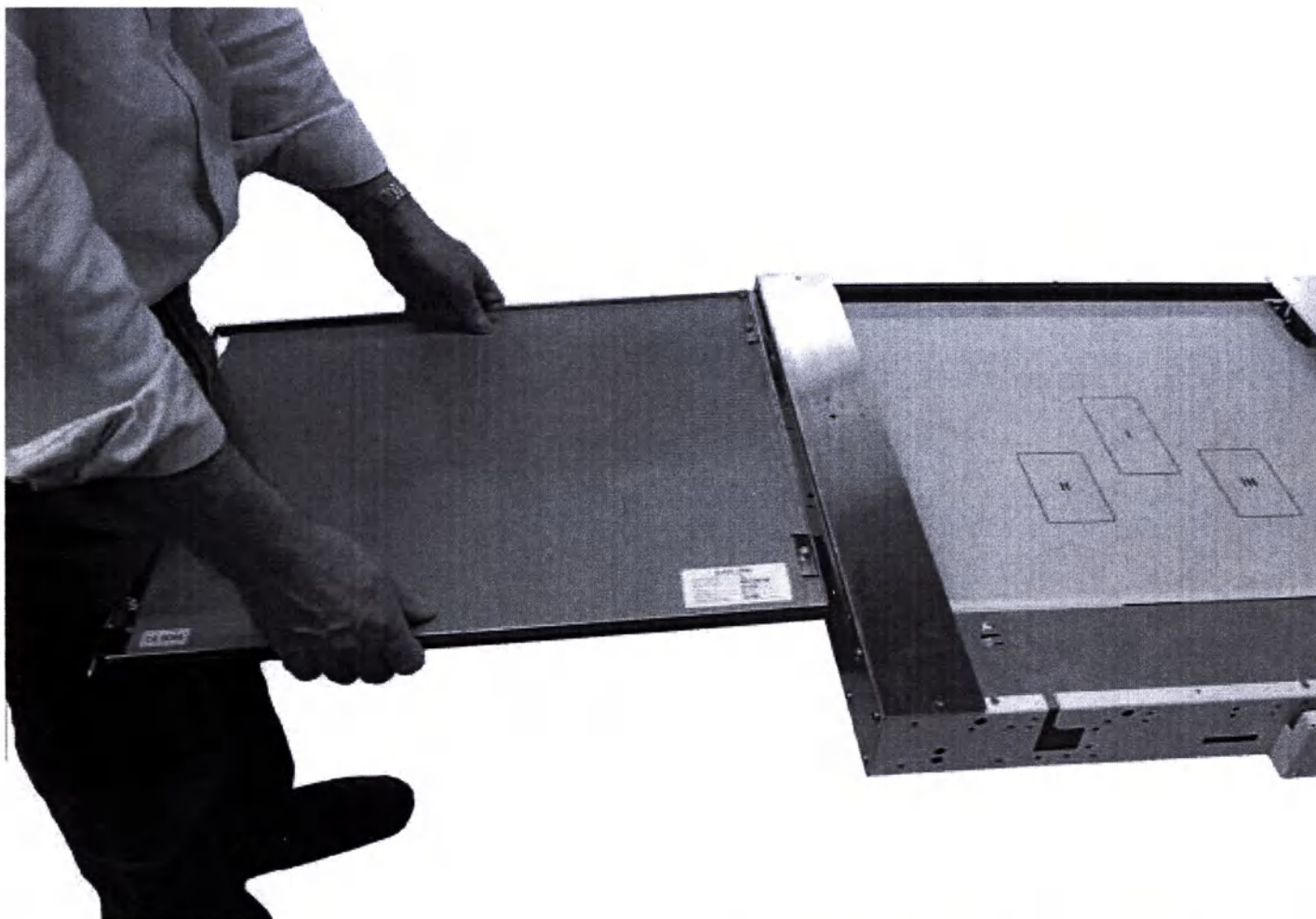
Отсеивающая фокусирующая решетка, система управления дозой АЕС, устройство букки
