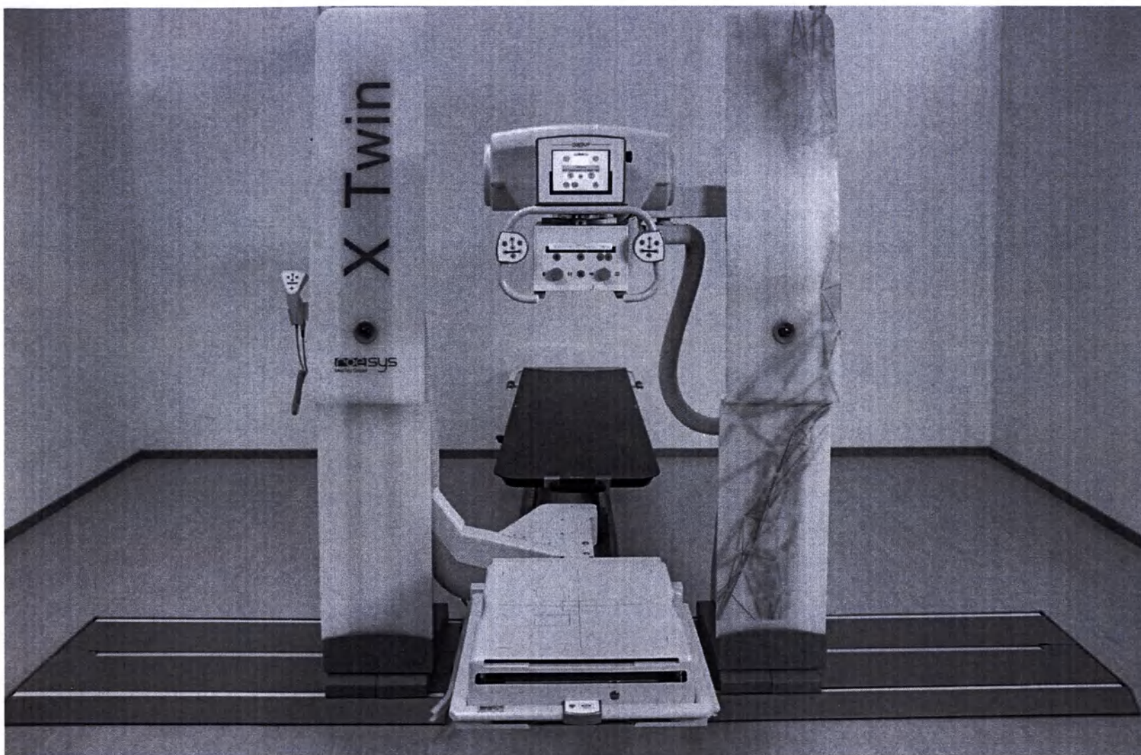
Колонна приемника изображения, основание колонны приемника изображения, колонна рентгеновского излучателя, основание колонны рентгеновского излучателя
