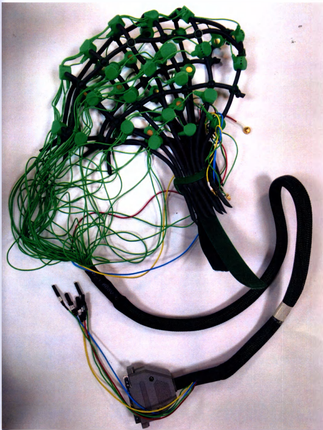
Шапка электродная Pamel КОМБИ ЭЭГ с предустановленными электродами Au
