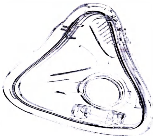
Уплотнители, корпуса дыхательных масок ResMed разноразмерные – XS, S, M, L, LW, XL, W, St
