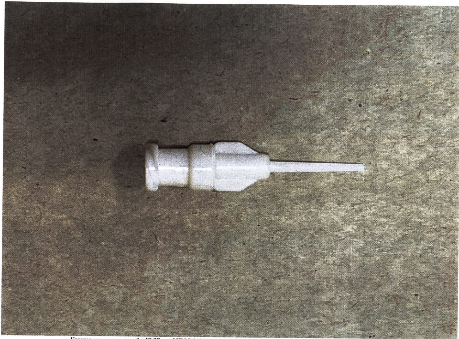
Катетер мочеточниковый «ЮЛЕ» по МПФР.942516.003 ТУ. Замок Луера для катетера размером: 5 Fr; 6 Fr; 7 Fr; 8 Fr
