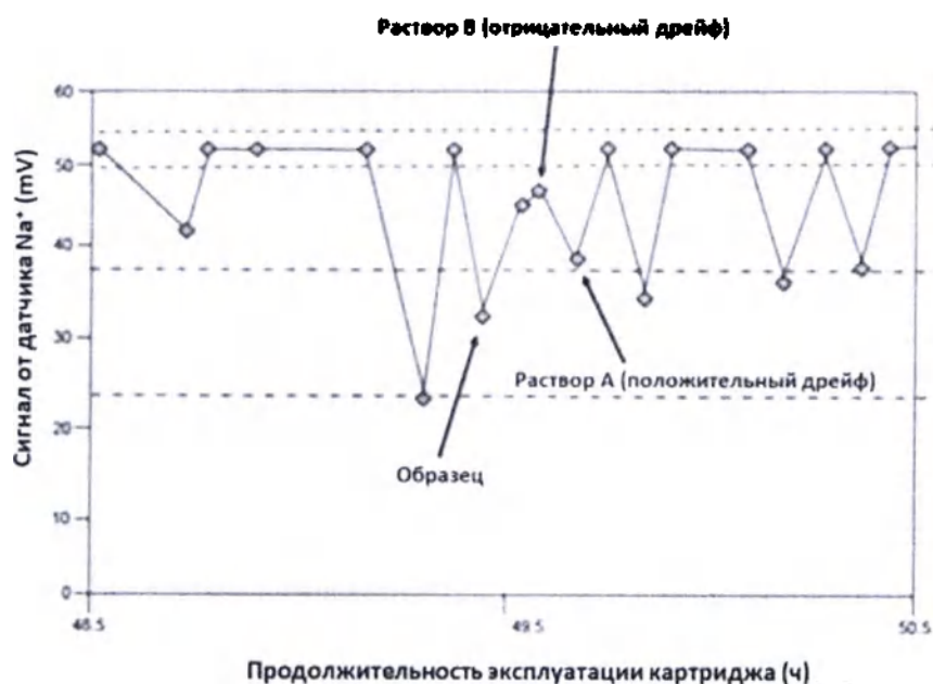
Рисунок 2с. Обнаружение микросдвигов: Отрицательный дрейф датчика по контрольному раствору В (PCS B) с последующим положительным дрейфом датчика по раствору А (PCS A).
