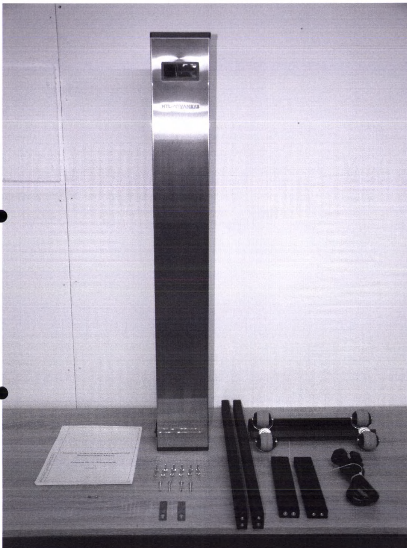
Облучатель - рециркулятор воздуха ультрафиолетовый бактерицидный «HTL-Advansys-30M»
