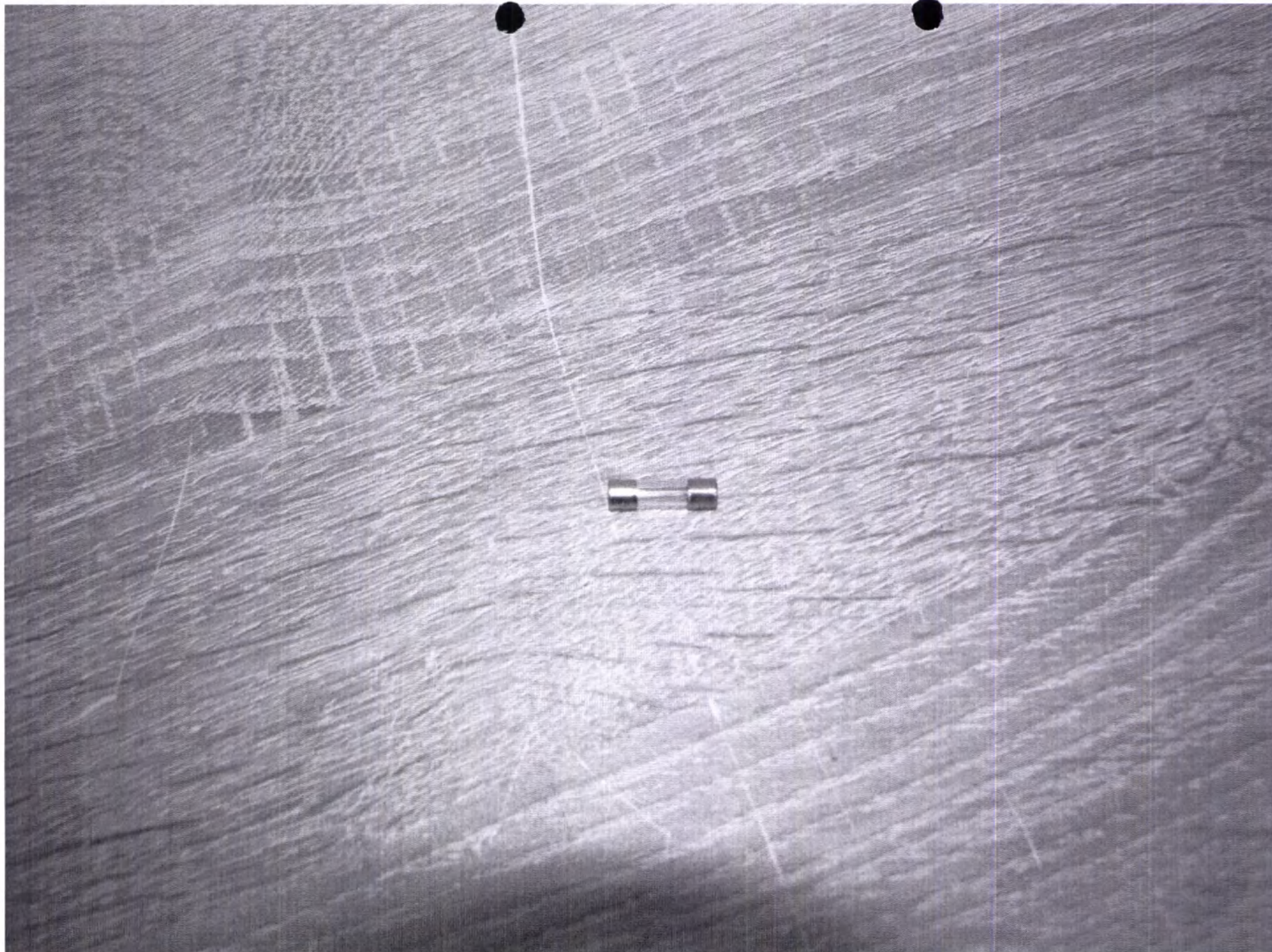
Предохранитель плавкий ВПБ6-11 3,15А 250 В, 5×20
