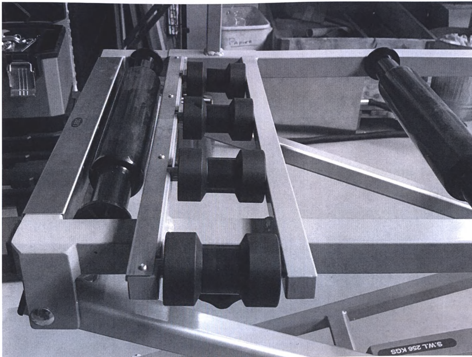
Рисунок 20 Съемные адаптеры для боковой загрузки лотка
