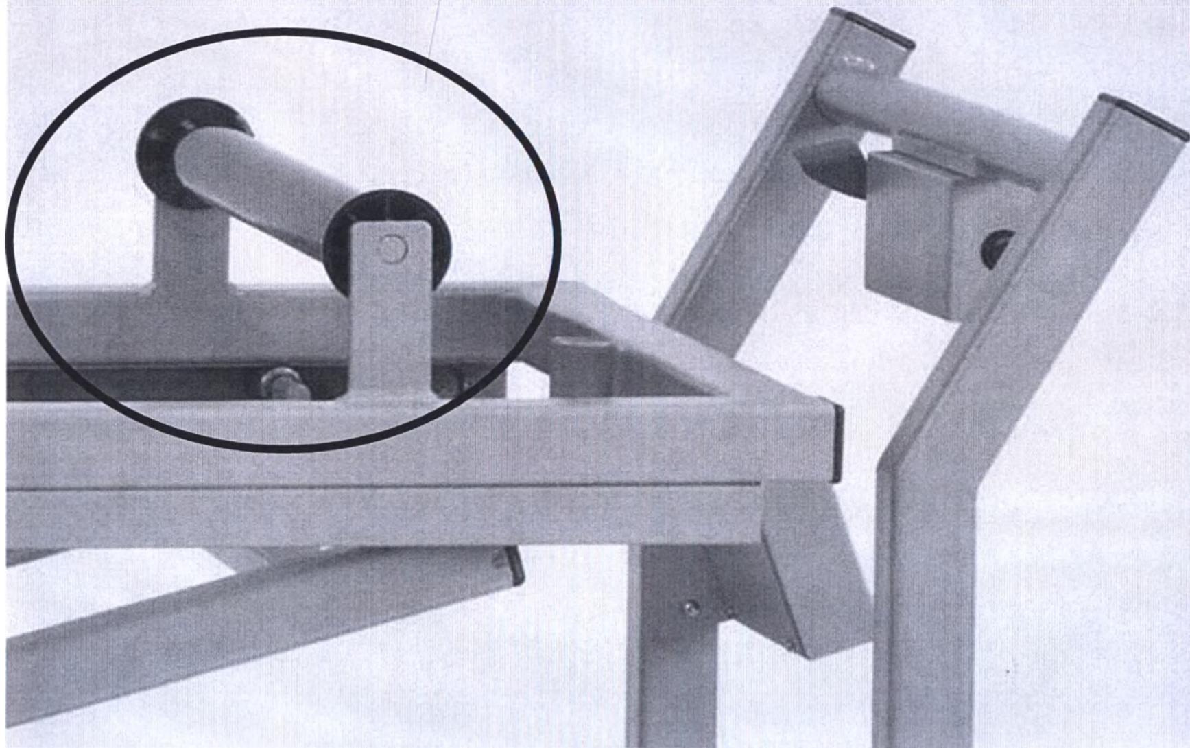
Рисунок 16 Поднятые ролики для лотка (при необходимости)
