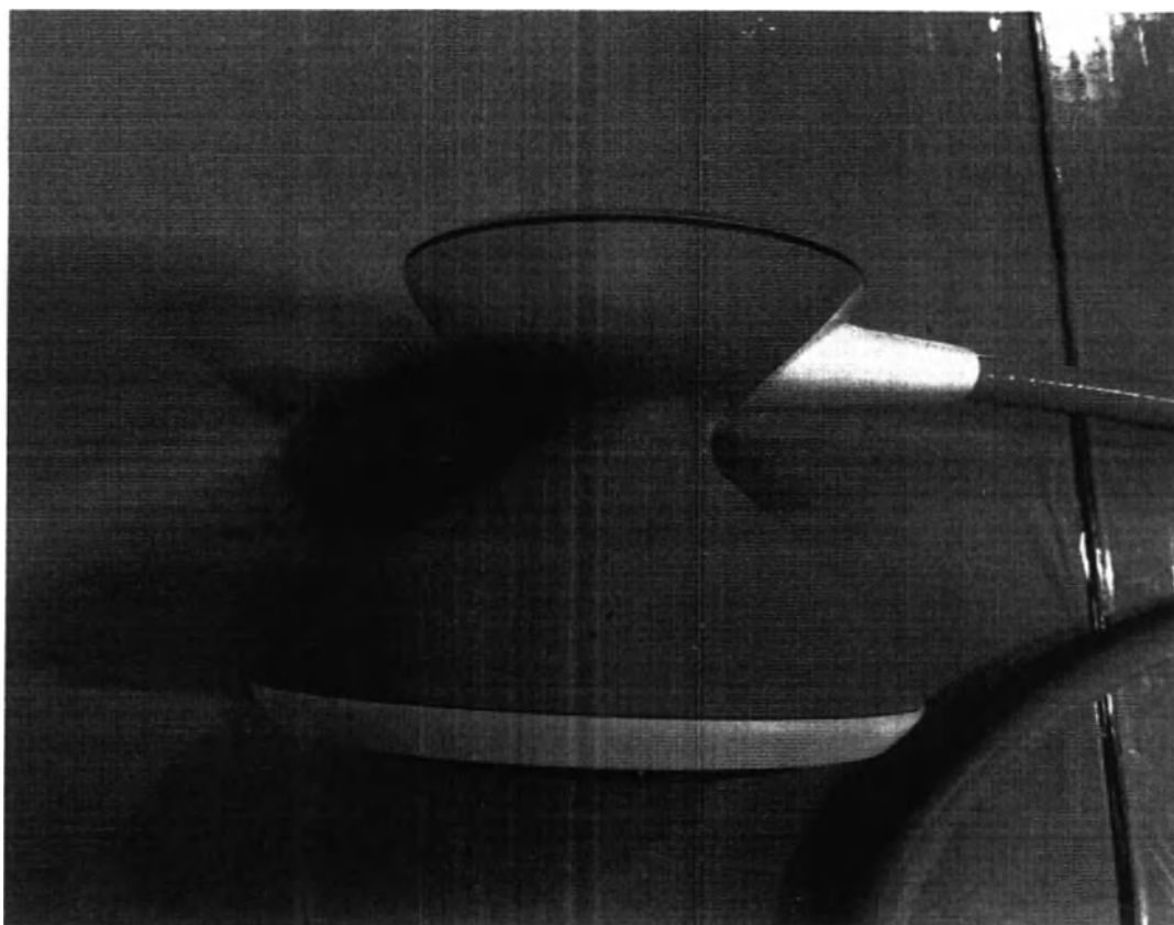
Аппликатор фокусированной ударно-волновой терапии
