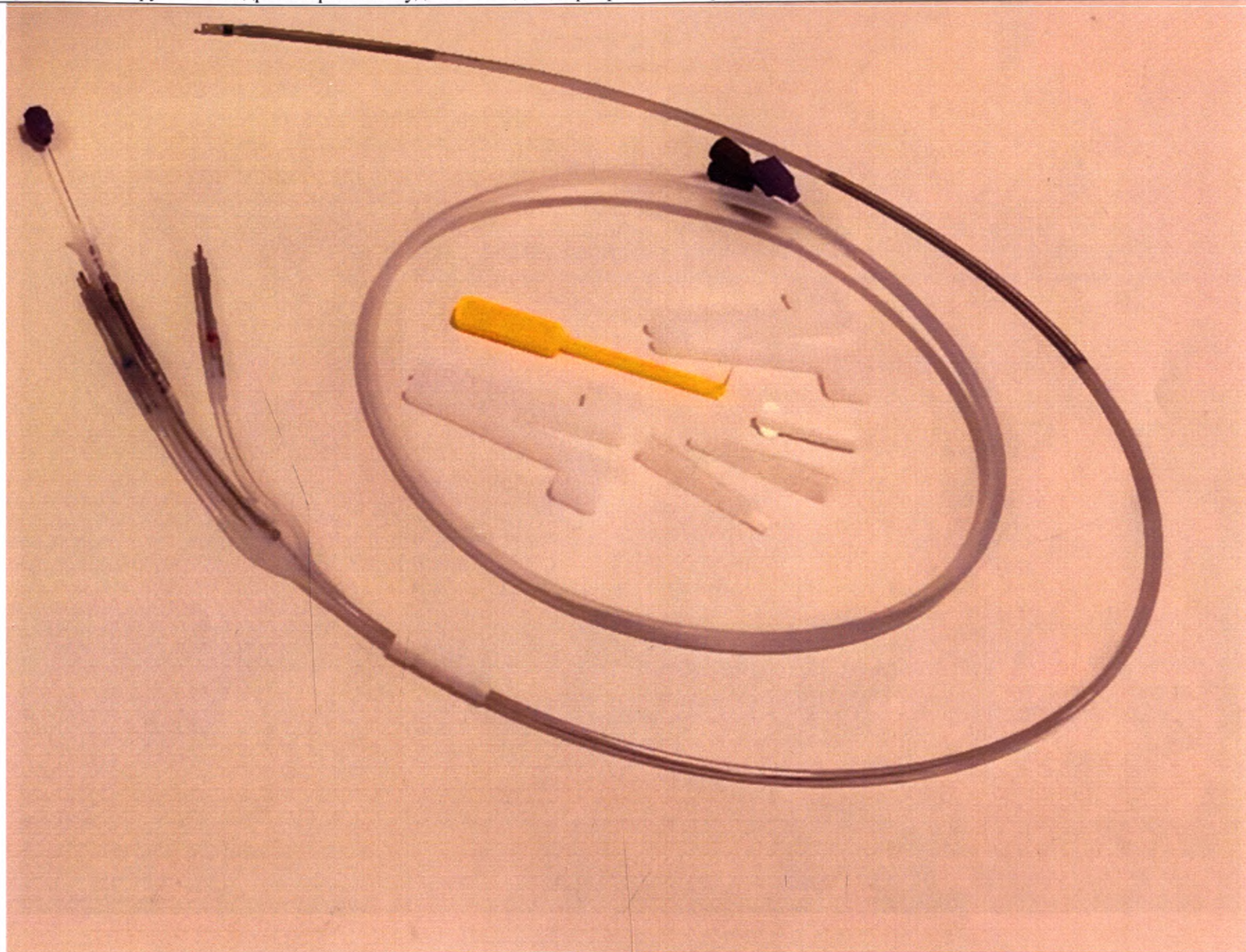
Электрод имплантируемый квадрополярный желудочковый для дефибрилляции Sprint Quattro Secure MRI Surescan 6947 на примере размера 65 см
