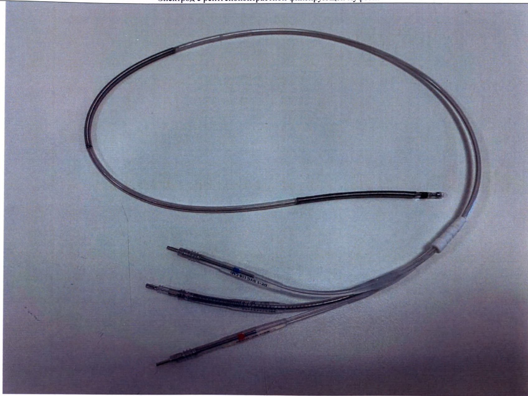
Электрод с рентгеноконтрастной фиксирующей муфтой.
