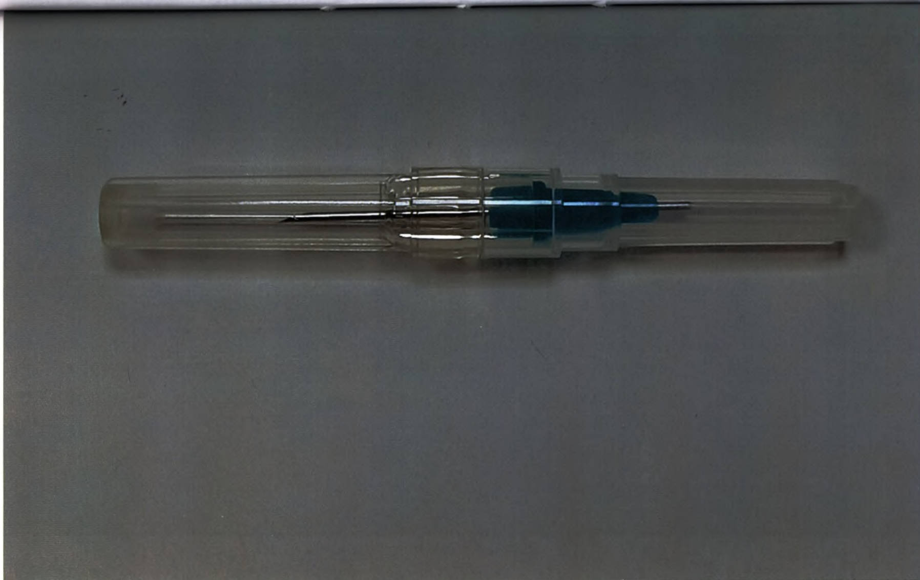
Рис 14. Микро-игла трубчатая, размер 21G x 3/4" (0,8 x 19 мм)
