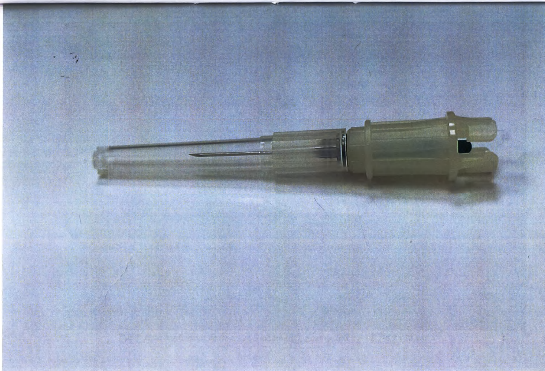
Рис 6. Игла трубчатая S-Monovette®, размер 22G x 1" (0,7 x 25 мм)
