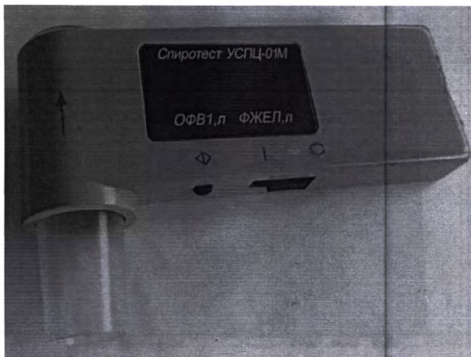
Рисунок 2 – Устройство мониторинга параметров внешнего дыхания человека, портативное цифровое «Спиротест УСПЦ-01М» по ТУ 26.60.12-003-18859607-2020, в составе с принадлежностями. Вид сзади
