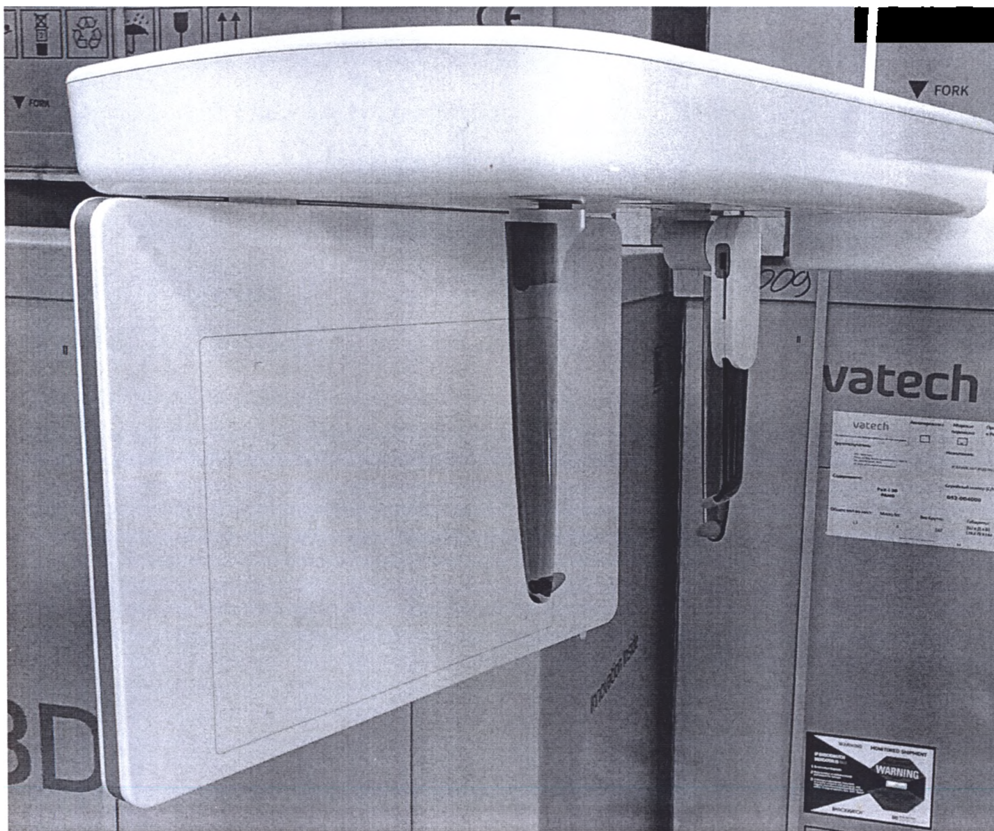
Цефалостат непрерывного сканирования с датчиком рентгеновского излучения цефалометрическим Xmaru2602CF
