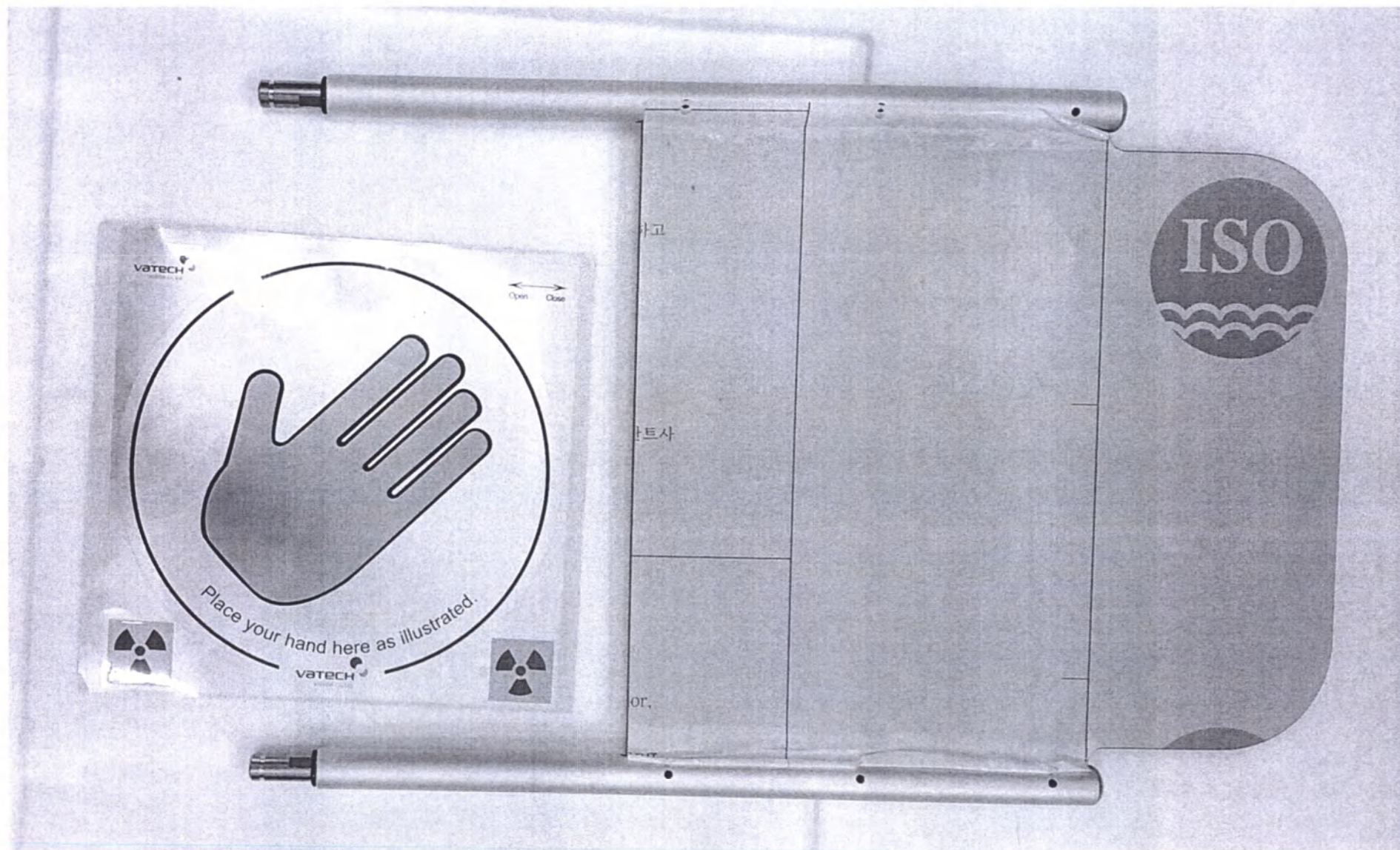
Позиционер запястья (справа) Наклейка позиционера запястья (слева)
