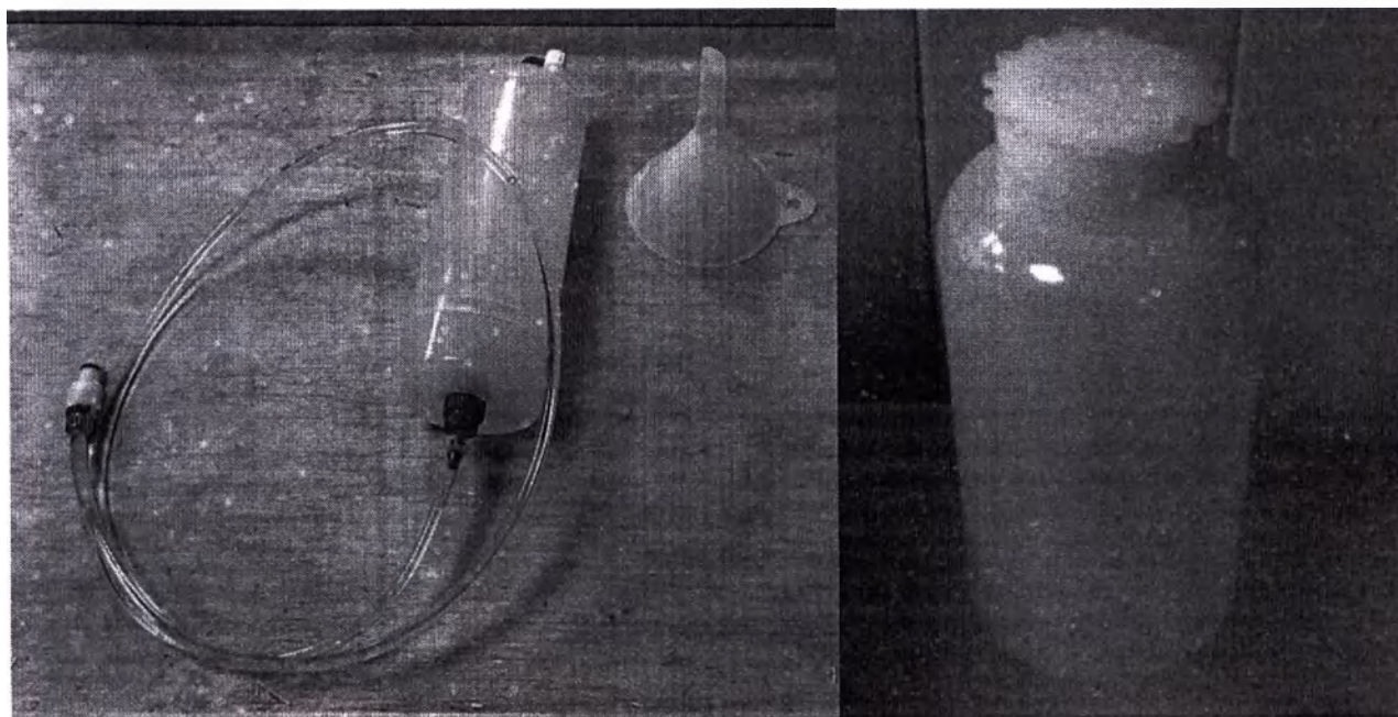
Комплект для заполнения системы охлаждения: Бутыль для заполнения и Шланг, Воронка, Жидкость охлаждающая для генератора
